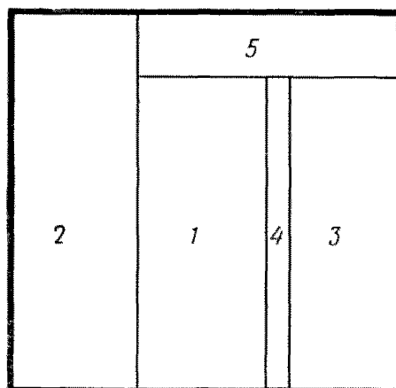
Рис. 53. Пример организации зоны отдыха в производственном корпусе завода радиоаппаратуры в г. Вестерос (Швеция)
