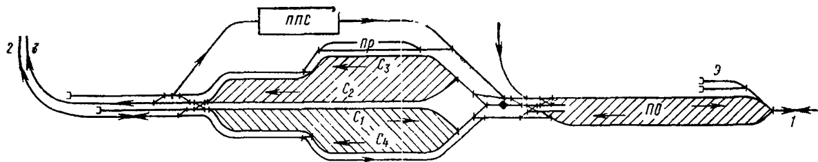
Рис. 31. Схема сортировочной станции нефтеперерабатывающего завода с последовательным расположением парков при кольцевой схеме путей, обслуживающих ТСБ C 1 — пути переработки вагонов для предприятий промзла; 3 — товарно-сырьевая база (остальные буквенные и цифровые обозначения те же, что для рис. 30)
