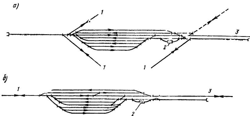
Рис. 11. Схемы грузовых станций
