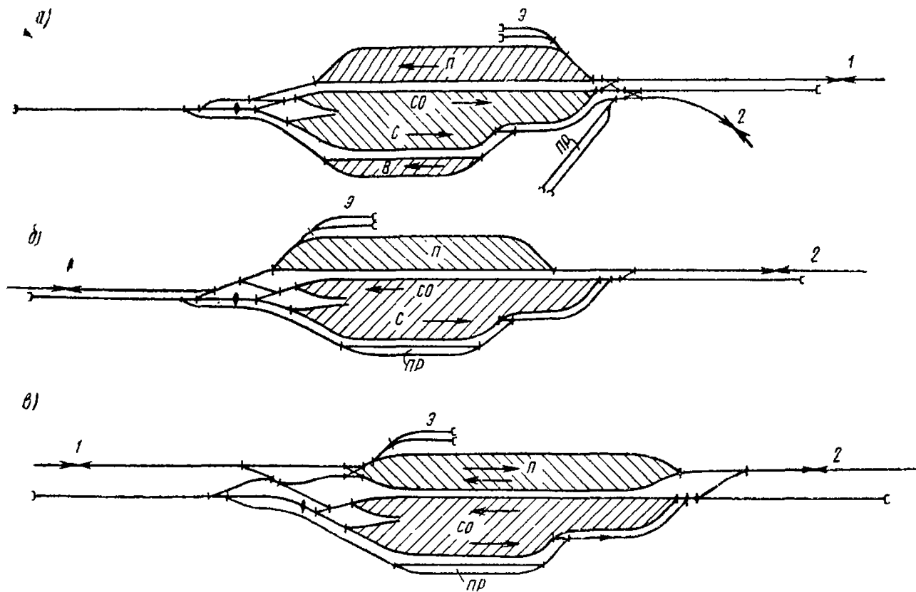
Рис. 24. Рекомендуемые схемы сортировочных станций с параллельным расположением парков a — с отдельными парками приема поездов с общей сети железных дорог ( П ) и подач с предприятий ( В ); б — с объединенным парком приема поездов и подач ( П ); в — со спускной частью горки, расположенной под углом к сортировочному парку; С — сортировочный парк; СО — сортировочно-отправочный парк; Э — пути пункта экипировки; ПР — пути отцепочного ремонта вагонов; 1 — станция примыкания; 2 — предприятия
