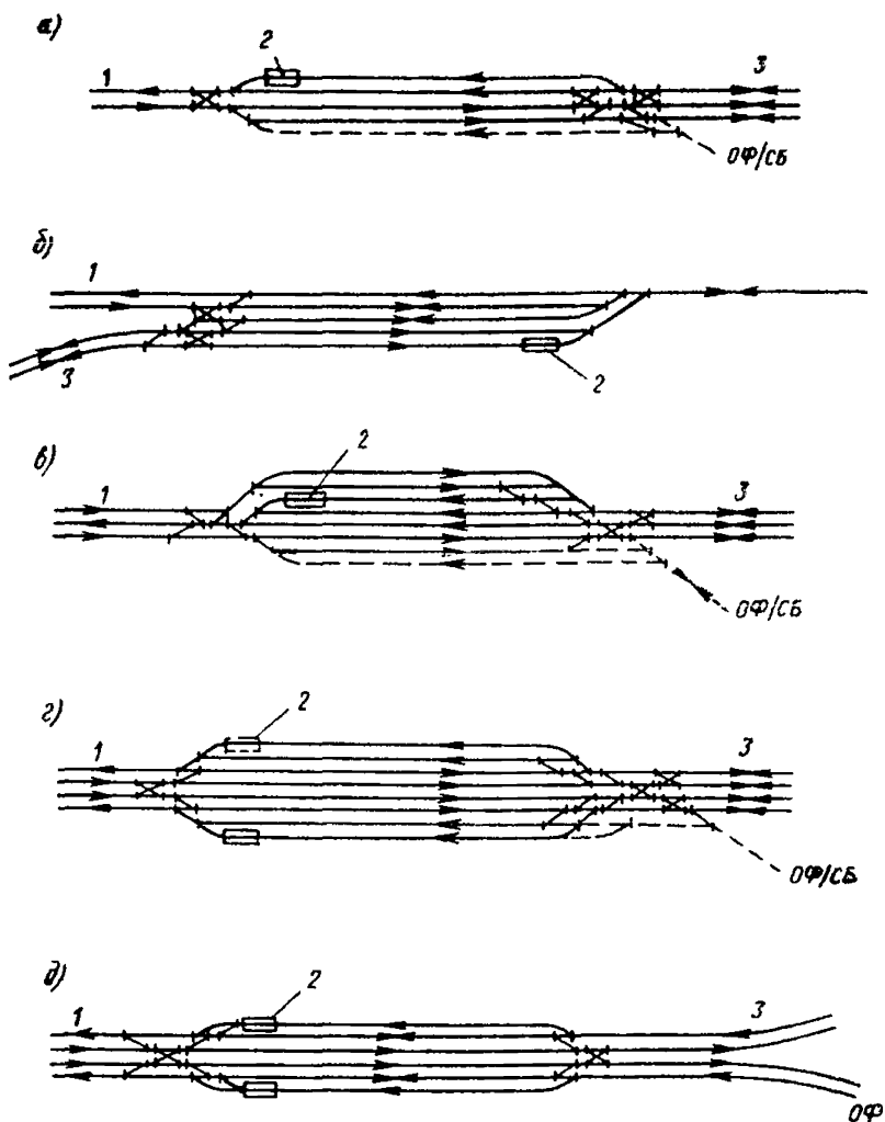
Рис. 10. Схемы карьерных распределительных станций а — при двухпутной выездной траншее; б — при двухпутной выездной траншее с угловым движением на отвал; в — при трехпутной выездной траншее; г — при четырехпутной выездной траншее; д — при четырехпутной выездной траншее и двухпутных подходах с отвалов и обогатительной фабрики; 1 — карьер; 2 — смотровая канава; 3 — отвалы
