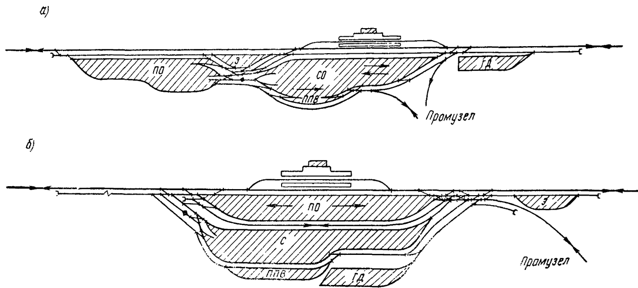
Рис. 48. Схемы грузовых станций на однопутных линиях при примыкании к ним подъездных путей
