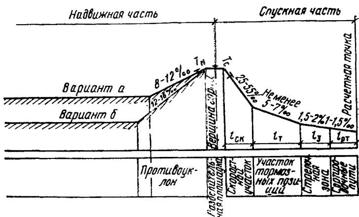
Рис. 40. Профиль горки малой мощности
