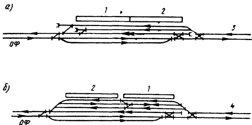
Рис. 34. Схемы углесборочных станций, не имеющих выхода на общую сеть железных дорог а — при движении из карьера с локомотивом в «хвосте» состава; б — при движении из карьера с локомотивом в «голове» состава; ОФ — обогатительная фабрика; 1 и 2 — положение составов, принимаемых из карьеров (шахт); 3 — карьер (шахты)
