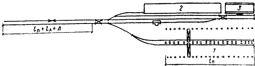
Рис. 4. Схема путей грузового пункта с линейными фронтами для разнородных грузов 1 — открытый склад с мостовыми кранами; 2 — закрытый склад; 3 — закрытый склад с рампой
