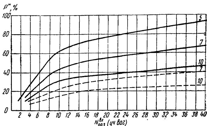
Рис. 53. График для определения вероятности появления в разборочном поезде вагонов с неоднородными грузами на грузовой фронт. Сплошная линия — при разборочном вагонопотоке от 400 до 600 учетных вагонов в сутки; пунктирная линия — при разборочном вагонопотоке от 800 до 1200 учетных вагонов в сутки; цифры 5, 7 и 10 — число разборочных поездов.
