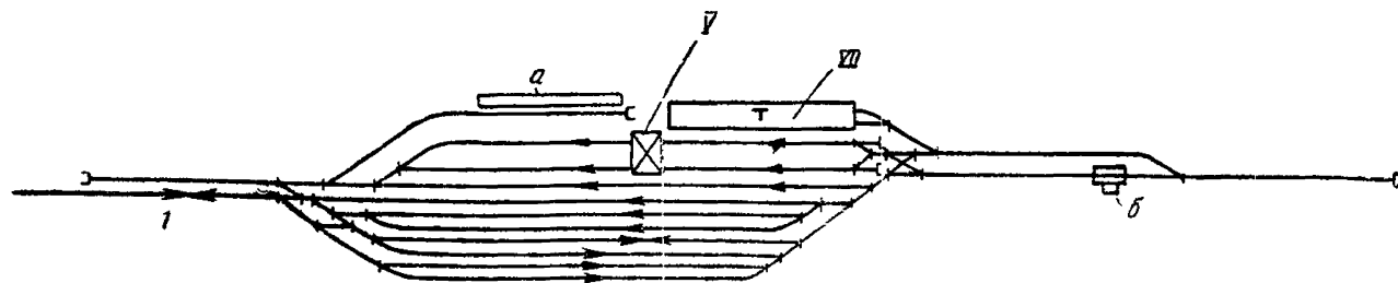
Рис. 15. Схема железнодорожной станции тепловой электростанции 1 — станция примыкания; а — эстакада слива жидкого топлива; б — весы (обозначения сооружений те же, что на рис. 2)
