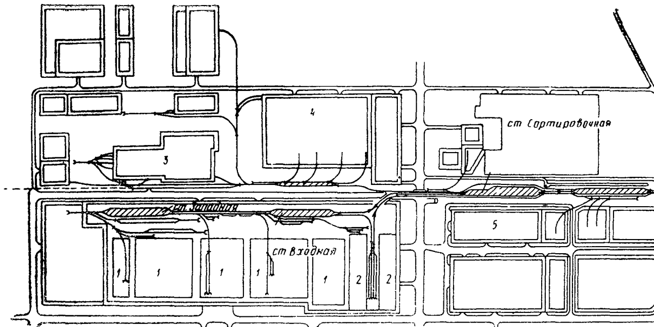
Рис. 22. Схема размещения сортировочной станции в увязке с генеральным планом промышленного узла машиностроительного профиля 1 — машиностроительный завод; 2 — погрузочная площадка машиностроительного завода; 3 — ТЭЦ; 4 — строительная база; 5 — завод пластмасс
