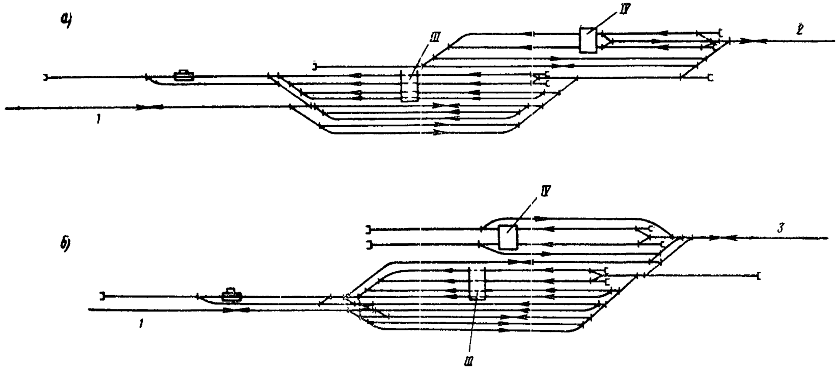
Рис. 12. Схемы углегрузочных станций при прибытии угля в саморазгружающихся вагонах предприятий а — прибытие с локомотивом в «голове» состава; б — прибытие с локомотивом в «хвосте» состава; 1 — станция примыкания; 2 — шахты; 3 — карьеры (обозначения сооружений те же, что на рис. 2)
