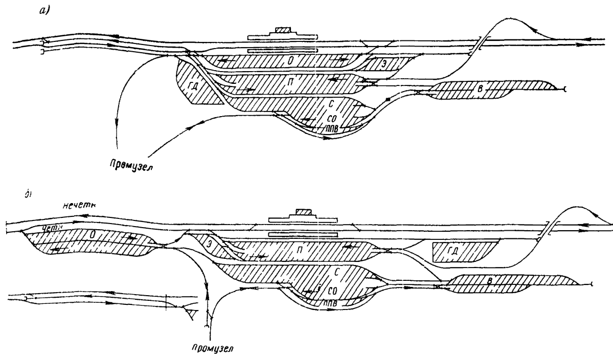
Рис. 50. Схемы объединенных станций на двухпутных линиях с промышленными парками при расположении парков станций по одну сторону главных путей
