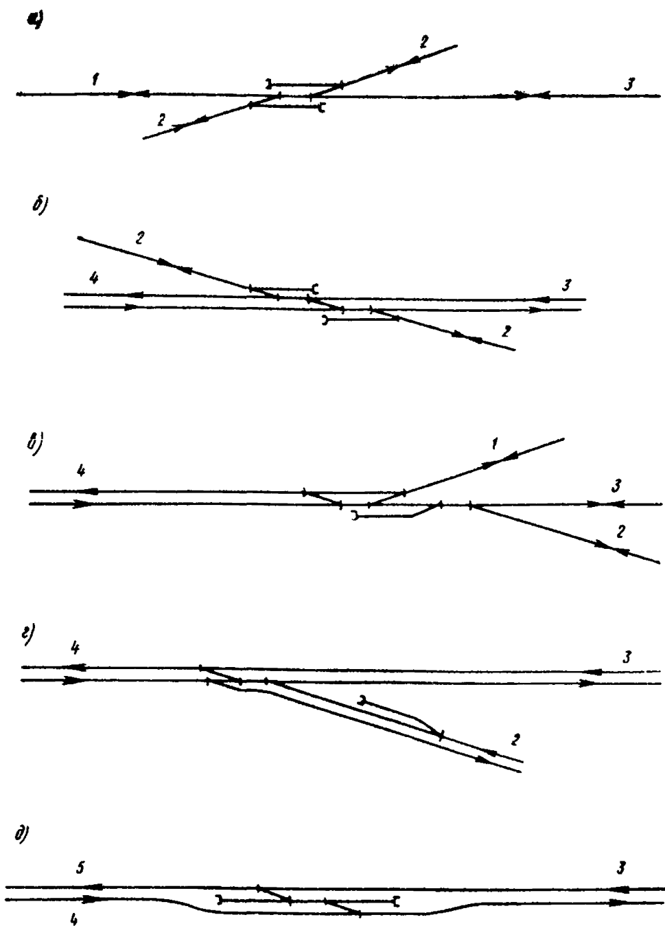
Рис. 7. Схемы постов примыкания к откаточным путям в карьерах a — примыкание путей к однопутному участку; б — примыкание путей к двухпутному участку; в — слияние однопутных участков в двухпутный участок; г — слияние двух двухпутных участков; д — пост шлюзового типа для толкачей; 1 — верхний горизонт; 2 — нижний горизонт; 3 — горизонт; 4 — въездная траншея; 5 — участок подталкивания
