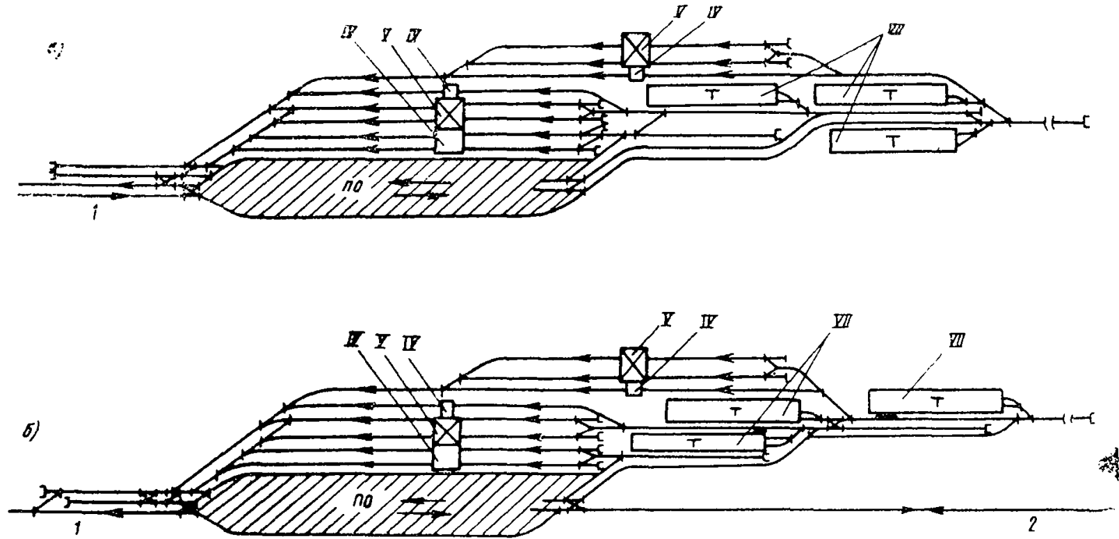
Рис. 16. Схема сырьевых станций металлургических заводов а — тупиковая; б — сквозная; 1 — сортировочная станция, завод; 2 — станция примыкания (обозначения сооружений те же, что на рис. 2)
