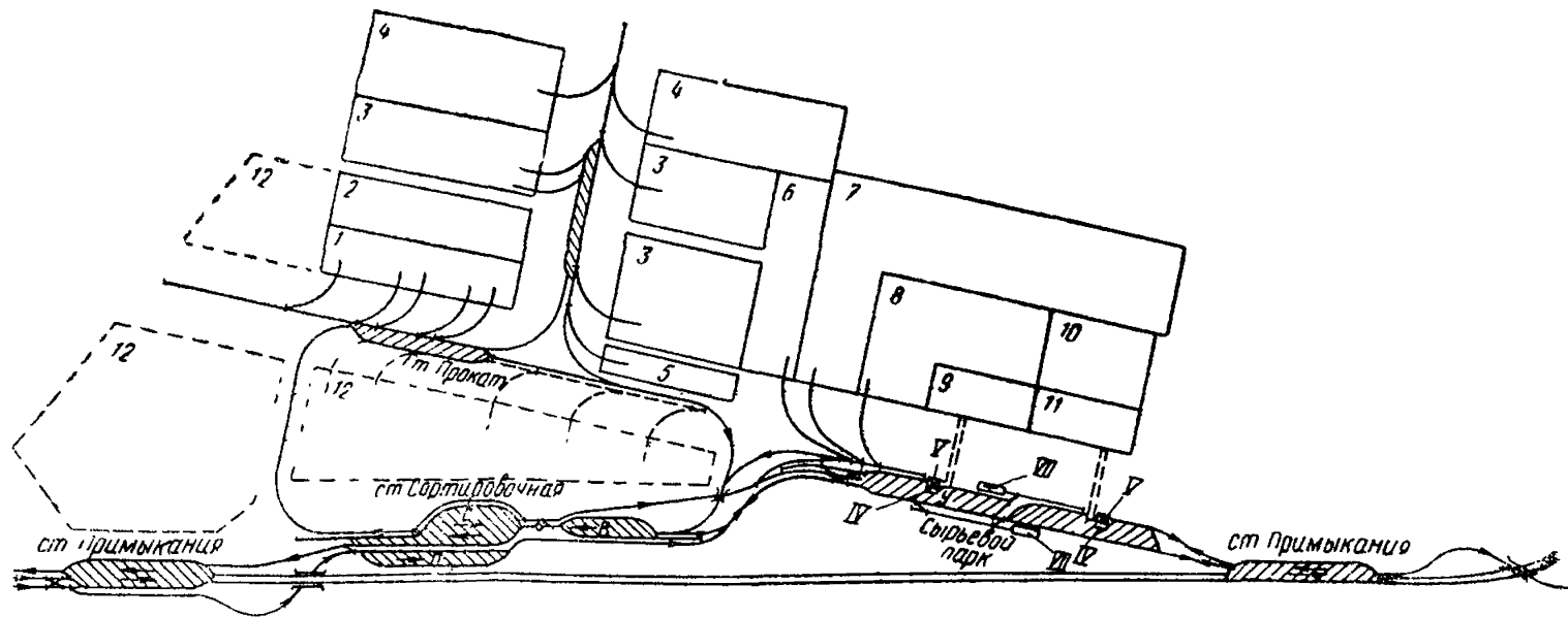
Рис. 19. Схема размещения сортировочной станции в увязке с генеральным планом металлургического завода П — парк приема; С — сортировочный парк; В — выставочный (предгорочный) парк; У — угольный парк; Р — рудный парк; 1 — складское хозяйство; 2 — ремонтные цехи; 3 — прокатные цехи; 4 — трубные цехи; 5 — скрапное хозяйство; 6 — сталеплавильный цех; 7 — доменный цех; 8 — коксохимический цех; 9 — склад угля; 10 — аглофабрика; 11 — склад руды; 12 — резервные территории (обозначения сооружений те же, что на рис. 2)
