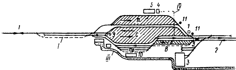
Рис. 39. Схема размещения сооружений и устройств на сортировочной станции с параллельным расположением парков (цифровые обозначения те же, что на рис. 37)
