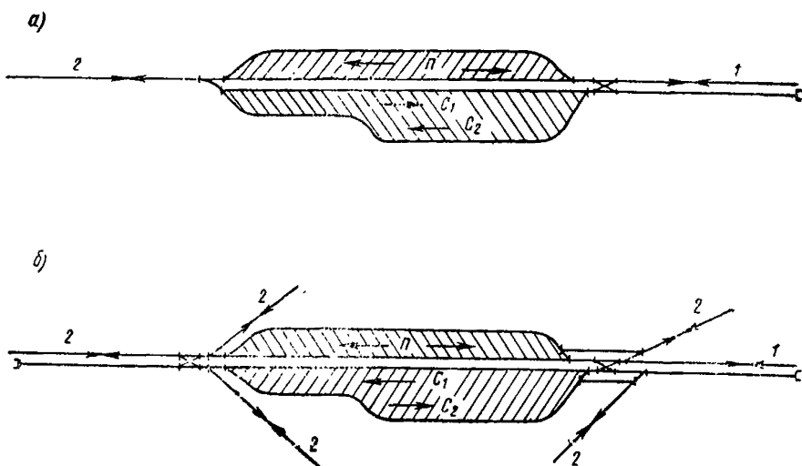
Рис. 25. Схемы безгорочных сортировочных станций а — при расположении перед предприятиями; б — при расположении между предприятиями; П — парк приема; С 1 — пути сортировки в направлении общей сети железных дорог; С 2 — пути сортировки в направлении предприятий; 1 — станция примыкания; 2 — предприятия
