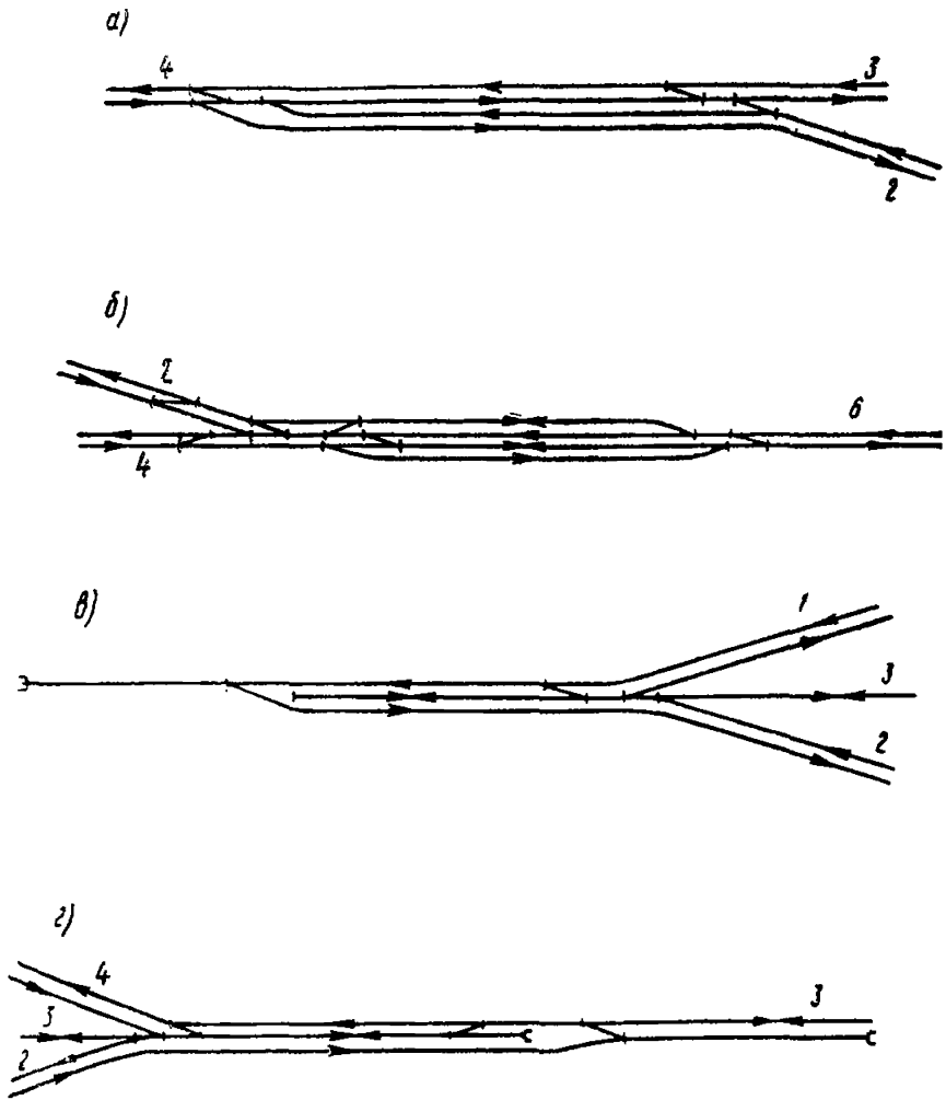
Рис. 9. Схемы постов слияния двухпутных участков с путевым развитием (в карьерах) а — слияние двух двухпутных участков; б — слияние двух двухпутных участков с угловым заездом; в — тупиковый телескопический пост; г — телескопический пост; б — на горизонт (остальные цифровые обозначения те же, что на рис. 7)
