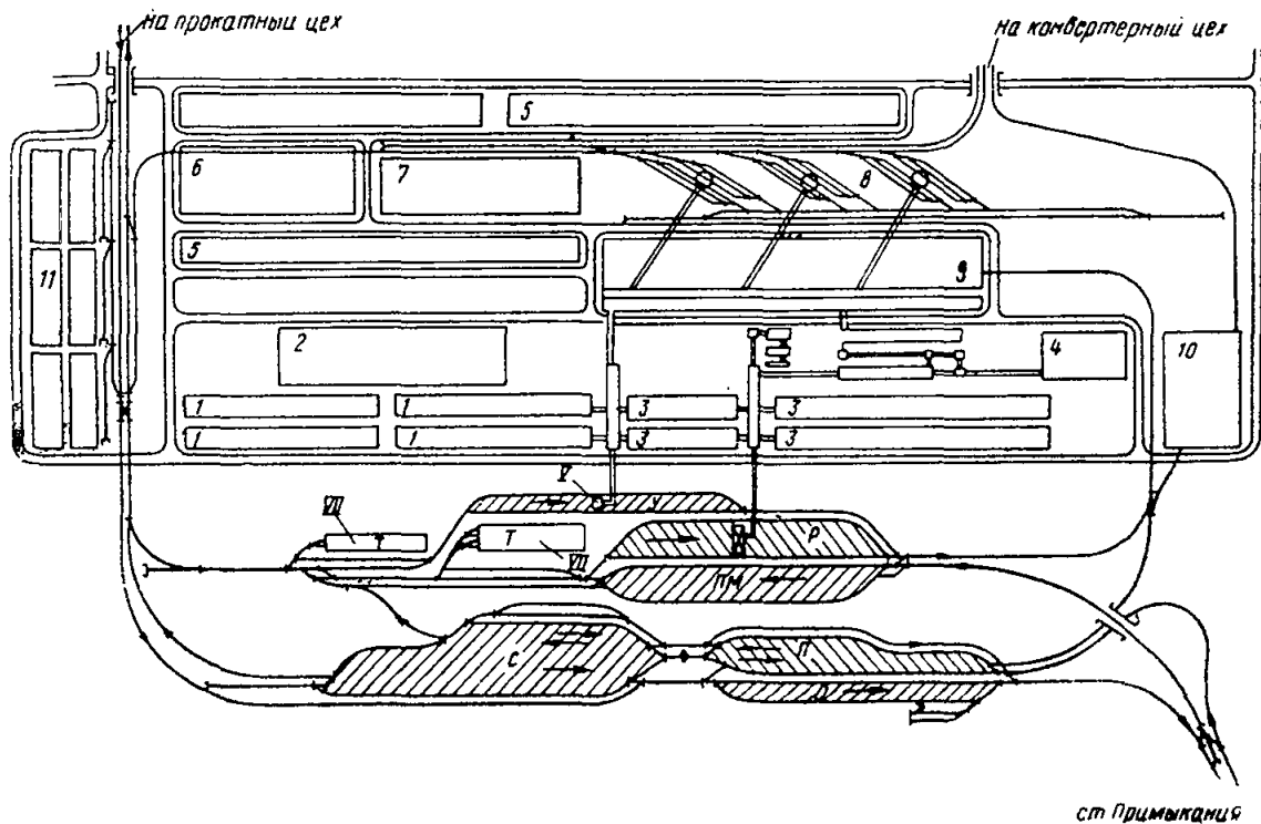
Рис. 28. Схема сортировочной станции, расположенной параллельно металлургическому заводу (на одной площадке с сырьевым парком)
