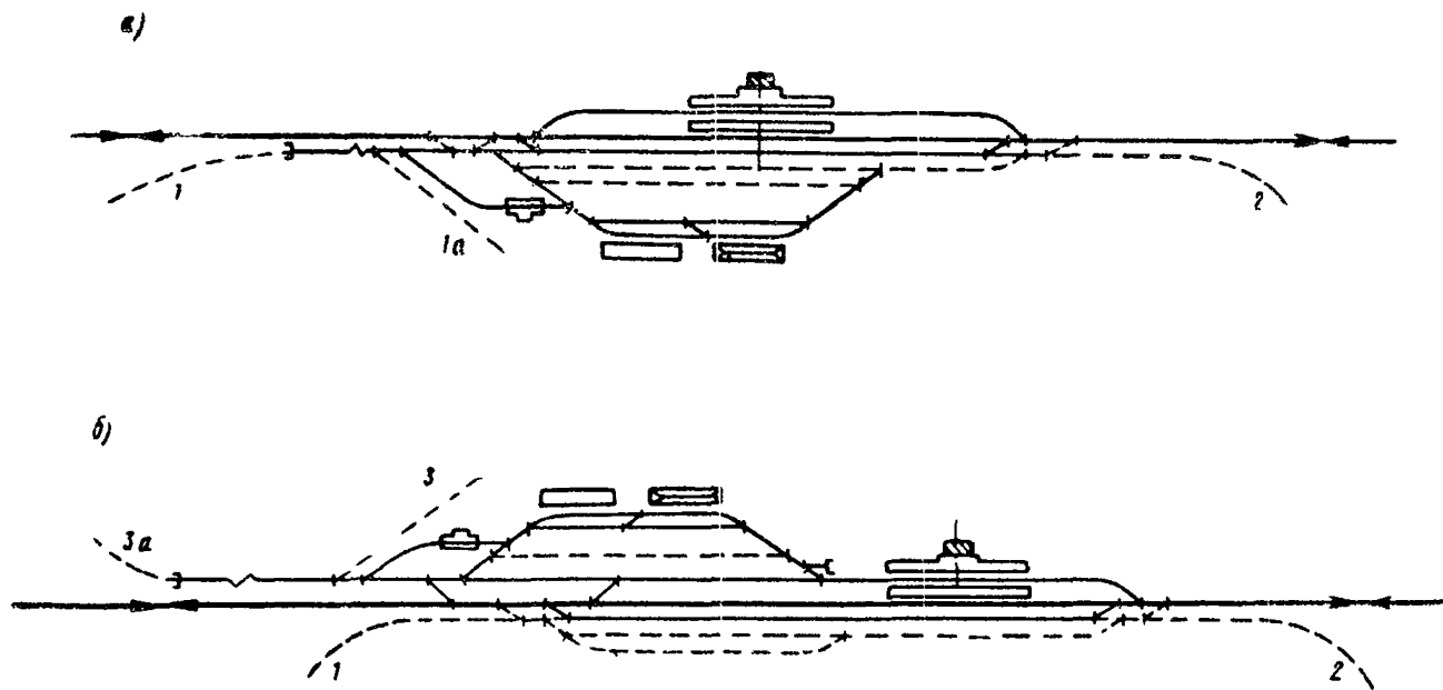
Рис. 44. Схемы промежуточных станций поперечного типа на однопутных линиях при примыкании к ним подъездных путей 1, 1а, 2, 3, 3а — варианты примыкания
