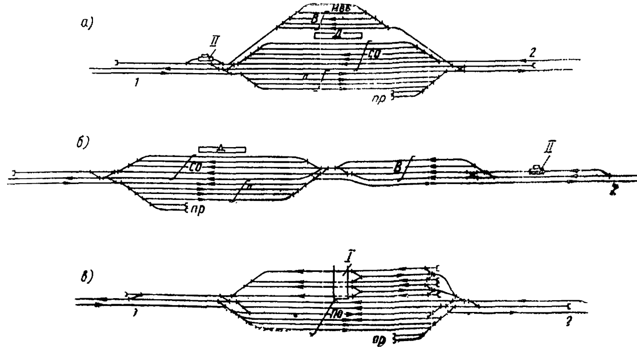
Рис. 35. Схемы углесборочных станций, отправляющих уголь на общую сеть железных дорог а — при взвешивании на станции вагонов с углем; б — при взвешивании вагонов с углем на подходе к станции на весах, допускающих пропуск локомотивов; в — при сплошной дозировке вагонов; МВБ — механизированная выгрузочная база; Д — дозировочные устройства; П — парк приема; ПО — приемо-отправочный парк; СО — сортировочно-отправочный парк; В — выставочный парк; ПР — пути отцепочного ремонта вагонов; I — погрузочное устройство; II — вагонные весы; 1 — станция примыкания; 2 — карьер (шахта) (рис. а) и карьер (рис. б и в)
