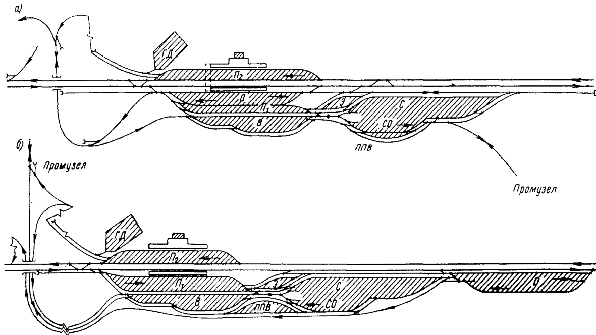
Рис. 4Ф. Схемы объединенных станций на двухпутных линиях с промышленными парками при расположении парков станции по обе стороны главных путей
