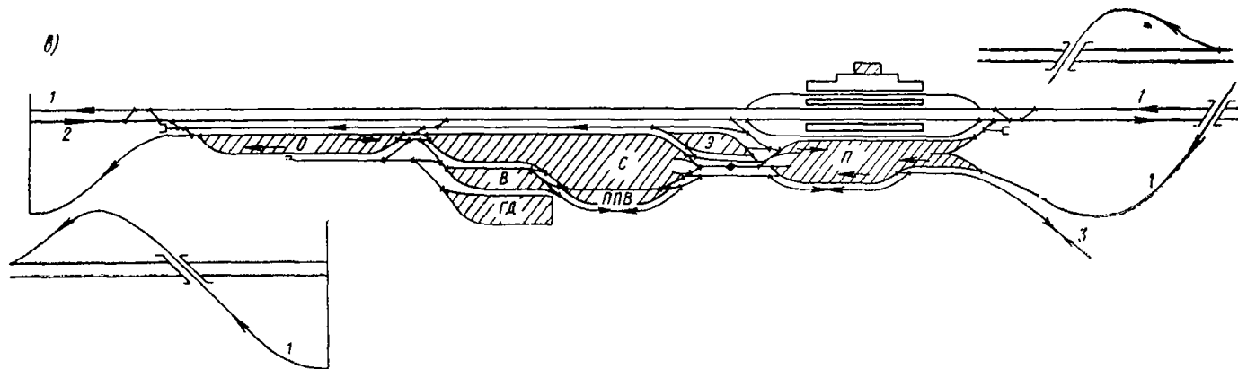
Рис. 47. Схемы грузовых станций на двухпутных линиях при примыкании к ним подъездных путей ГД — грузовой двор; направления движения: 1 — нечетное; 2 — четное; 3 — промузел
