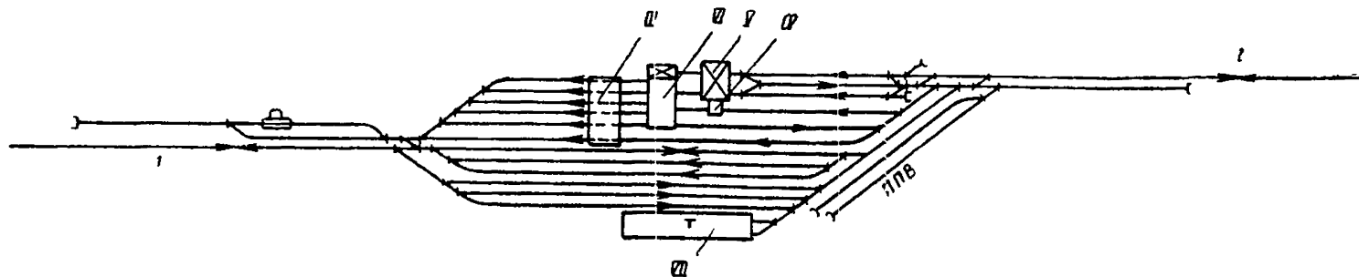
Рис. 14. Схема углепогрузочной станции при прибытии угля с общей сети железных дорог и местных шахт в полувагонах и использовании для расстановки вагонов при погрузке траверсной тележки 1 — станция примыкания; 2 — шахты; ППВ — пункт подготовки вагонов (обозначения сооружений те же, что на рис. 2)
