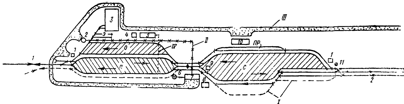
Рис. 37. Схема размещения сооружений и устройств на сортировочной станции с последовательно расположенными парками приема и отправочного железной дороги общей сети
