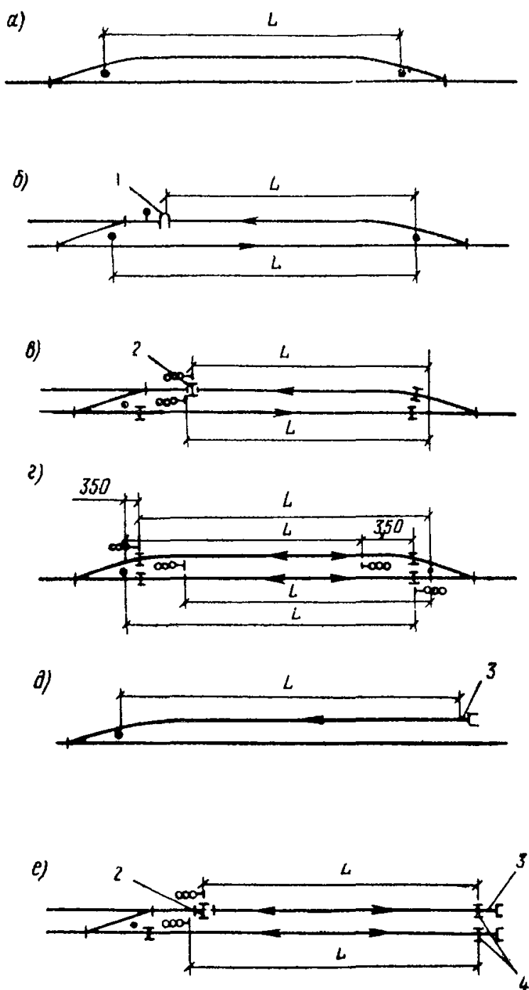
Рис. 1. Полезная длина станционных путей с учетом расположения сигналов и изолирующих стыков 1 — стык рамного рельса; 2 — стык рамного рельса и изолирующий; 3 — начало балластной призмы; 4 — изолирующие стыки
