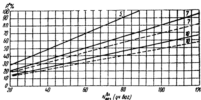
Рис. 54. График для определения вероятности появления в разборочном поезде вагонов с однородными грузами на грузовой фронт (значения сплошной и пунктирной линий, а также цифр 5, 7 и 10 те же, что на рис. 53)
