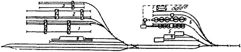
Рис. 18 Схема станции механизированной выгрузочной базы угольного района
