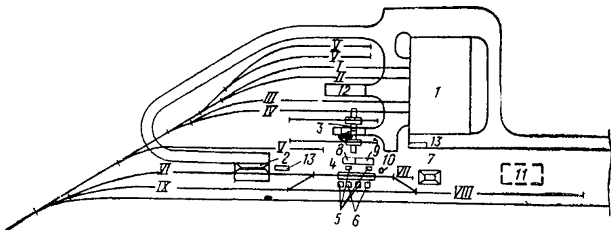
Рис. 36. Схема генерального плана при совместном размещении ремонтного хозяйства и экипировочных устройств
