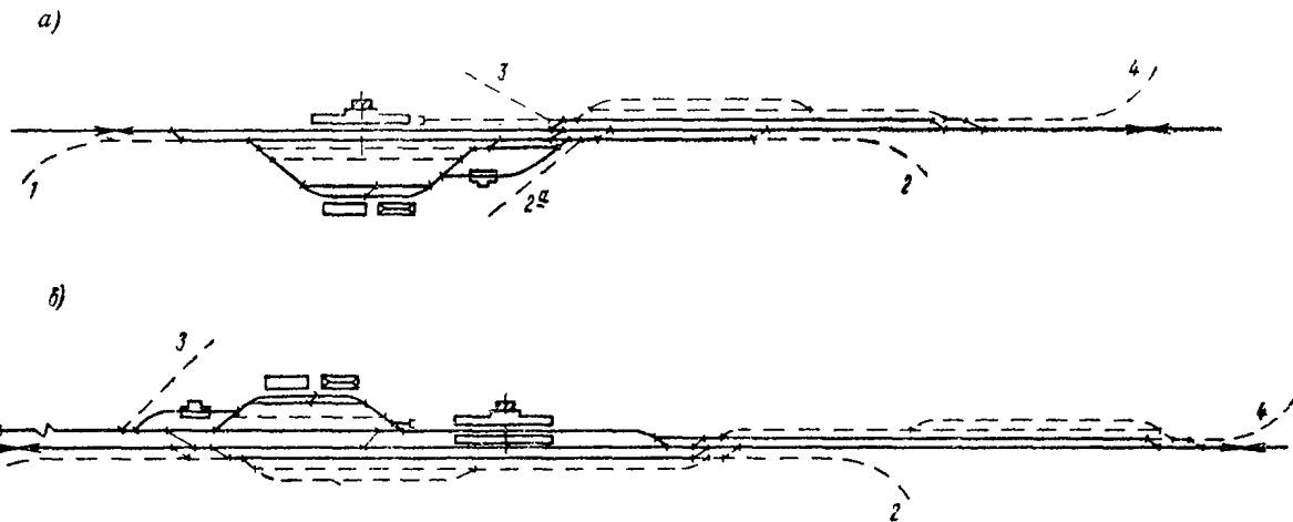
Рис. 45. Схемы промежуточных станций продольного типа на однопутных линиях при примыкании к ним подъездных путей 1, 2, 2а, 3, 4 — варианты примыкания
