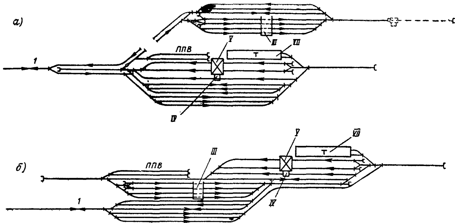
Рис. 13. Схемы углепогрузочных станций при прибытии угля с общей сети железных дорог в полувагонах а — расположение выгрузочных и погрузочных комплексов на отдельных площадках; б — расположение выгрузочных и погрузочных комплексов на общей площадке; 1 — станция примыкания; ППВ — пункт подготовки вагонов (обозначения сооружений те же, что на рис. 2)
