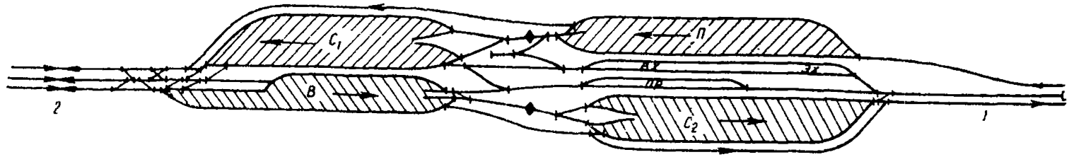
Рис. 29. Схема двухсторонней горочной сортировочной станции C_1 — сортировочный парк для расформирования входящего вагонопотока; C_2 — сортировочный парк для формирования поездов на общую сеть железных дорог; П — парк приема (предгорочный); В — выставочный парк; 1 — станция примыкания; 2 — предприятия
