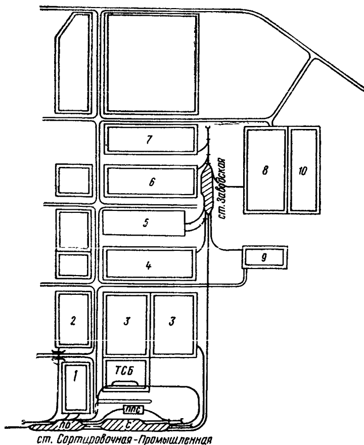
Рис. 21. Схема размещения сортировочной станции в увязке с генеральным планом промышленного узла нефтехимического профиля ПО — приемо-отправочный парк; С — сортировочный парк; ППС — промывочно-пропарочная станция; ТСБ — товарно-сырьевая база; 1 — завод железобетонных изделий; 2 — ремонтно-механический завод; 3 — нефтеперерабатывающий завод; 4 — завод пластмасс; 5 — ТЭЦ; 6 — азотно-туковый завод; 7 — хлорорганический завод; 8 — складская зона; 9 — завод асфальтобетонный; 10 — резервная площадка
