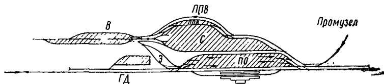
Рис. 51. Схема объединенной станции на однопутной линии с промышленными парками
