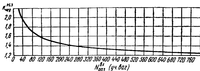
Рис. 52. График для определения суточного коэффициента неравномерности вагонопотоков
