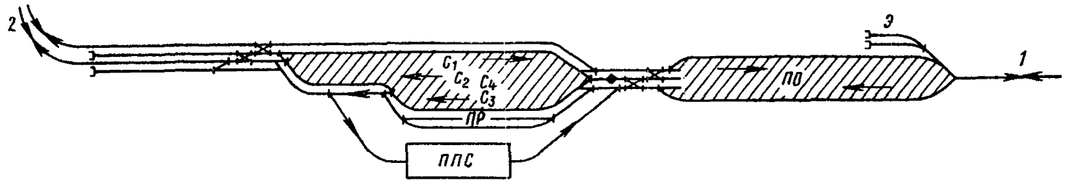
Рис. 30. Схема сортировочной станции нефтеперерабатывающего завода с последовательным расположением парков C_1 — пути формирования поездов на общую сеть железных дорог; C_2 — пути формирования составов под налив на ТСБ; C_3 — пути переработки вагонов для ППС и предприятий промзла; ПО — приемо-отправочный парк; 1 — станция примыкания; 2 — предприятия
