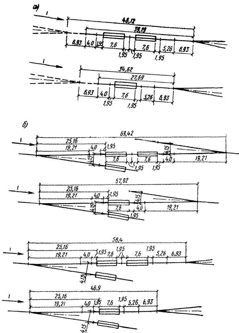
Рис. 41. Схемы расположения вагонных замедлителей типа KB3 на спусковой части сортировочных устройств а — на верхней тормозной позиции перед раздельной стрелкой; б — на нижней тормозной позиции после первой раздельной стрелки; 1 — направление роспуска
