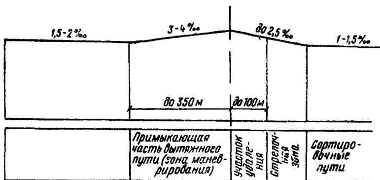
Рис. 43. Профиль вытяжного пути со стрелочной горловиной на уклоне
