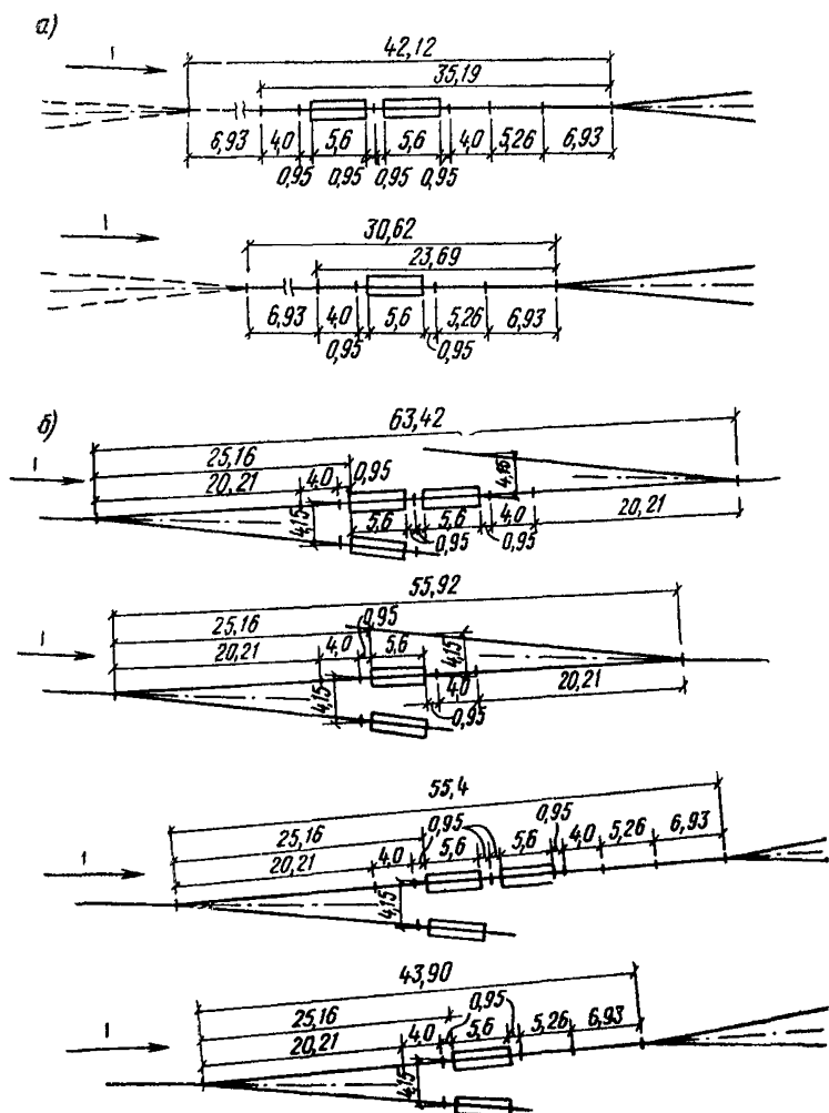
Рис. 42. Схема расположения вагонных замедлителей типа КВ2 на спускной части сортировочных устройств 1 — направление сортировки (позиции а и б те же, что на рис. 41)
