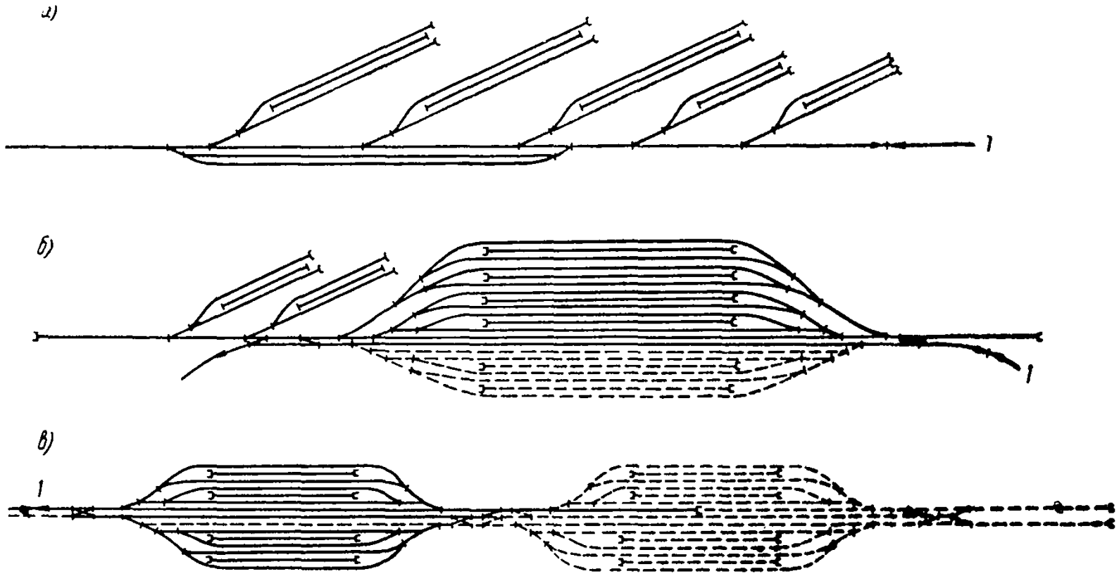
Рис. 17. Схемы нефтеналивных станций а — с туниковыми путями налива; б — с параллельным размещением эстакад; в — с последовательным размещением групп эстакад; 1 — подход с сортировочной станции
