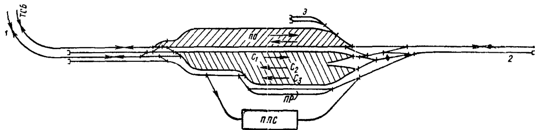
Рис. 32. Схема сортировочной станции нефтеперерабатывающего завода с параллельным расположением парков (буквенные и цифровые обозначения те же, что на рис. 30).
