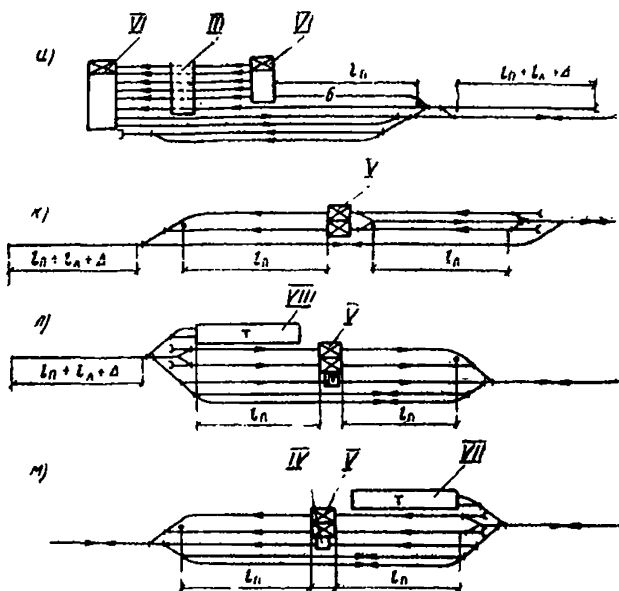
Рис. 2. Схемы грузовых пунктов с точечными фронтами l_n — длина подачи; l_l — длина локомотива; \Delta — неточность установки; I — бункерный склад с конвейерной подачей и выдачей материала; II — силосные склады; III — погрузочное устройство; IV — разгрузочное устройство; V — вагоноопрокидыватель; VI — траверзная тележка; VII — тепляк (размораживающее устройство)
