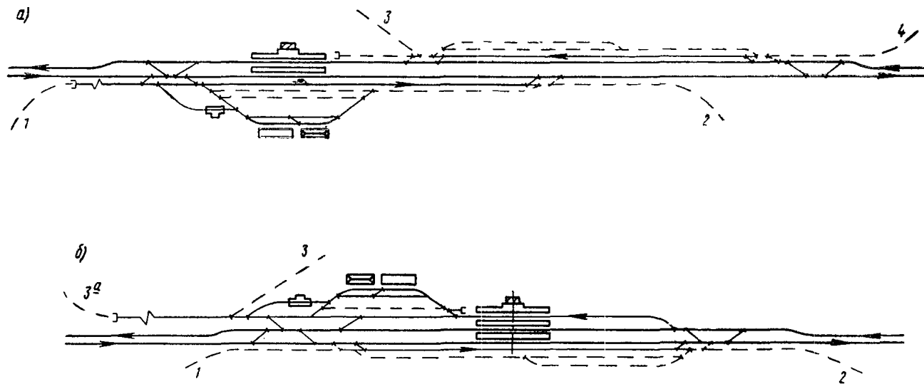
Рис. 46. Схемы промежуточных станций на двухпутных линиях при примыкании к ним подъездных путей
