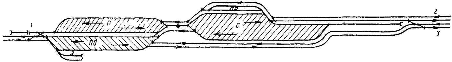
Рис. 26. Схема сортировочной станции, расположенной последовательно площадке металлургического завода П — предгорочный парк; ПО — приемо-отправочный парк; С — сортировочный парк; ПП — пути отцепочного ремонта вагонов; 1 — станция примыкания; 2 — завод; 3 — сырьевая станция
