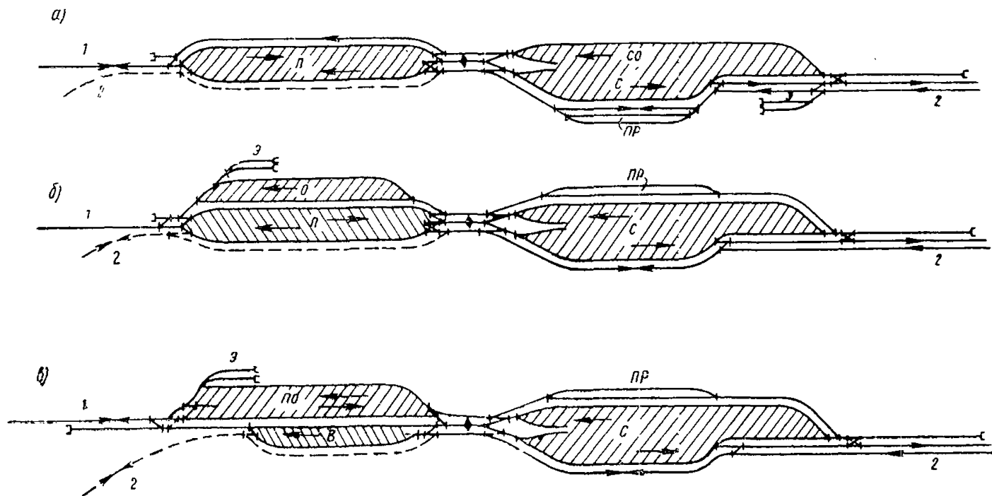
Рис. 23. Рекомендуемые схемы сортировочных станций с последовательным расположением парков а — с сортировочно-отправочным парком (СО); б — с отправочным парком МПС (О); в — с приемо-отправочным парком МПС (ПО); П — парк приема; С — сортировочный парк; В — выставочный парк; Э — пути пункта экипировки; ПР — пути отцепного ремонта вагонов; 1 — станция примыкания; 2 — предприятия
