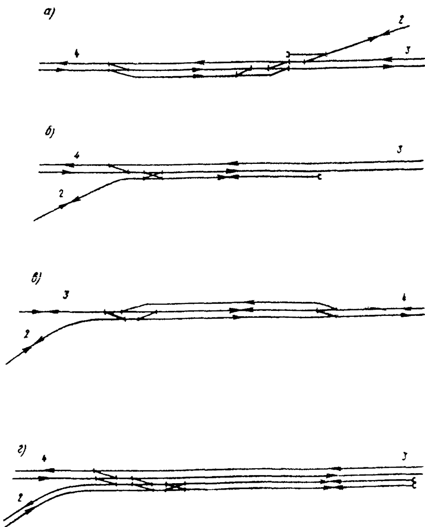
Рис. 8. Схемы постов с путевым развитием (в карьерах) а — попутное примыкание пути к двухпутному участку; б — примыкание пути к двухпутному участку с угловым заездом; в — слияние однопутных участков в двухпутный участок; г — примыкание двухпутного участка к двухпутному участку с угловым заездом (цифровые обозначения те же, что на рис. 7)
