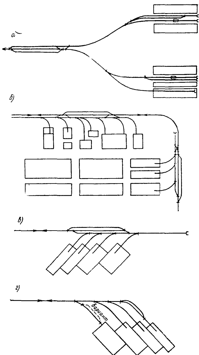
Рис. 5. Схемы размещения распределительных станций
