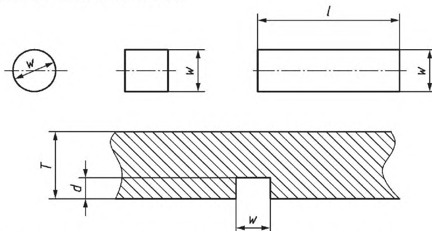
Рисунок 1 – Вид настроечных отражателей
