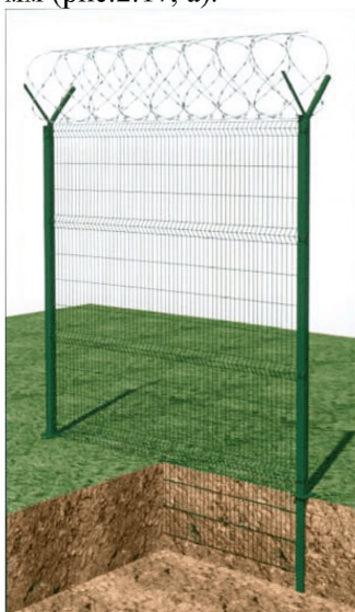
б) Заглубление сварной сетчатой панели
