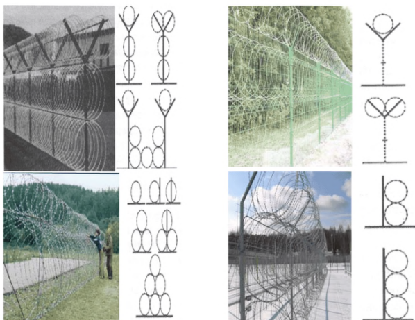
Рис. 2.10. Варианты комплексного использования оградений СББ и ПББ
