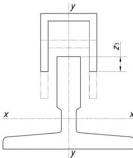
б) Минимальная требуемая длина перекрытия контрольного башмака во время землетрясения
