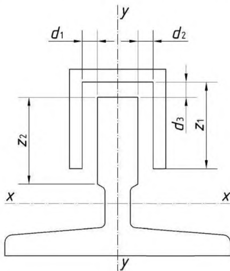
а) Номинальное положение и зазоры контрольного башмака
