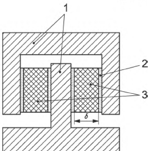
а) Измерение модуля Юнга
