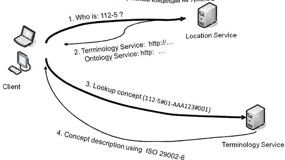
Рисунок 5 — Пример поиска концепций по идентификатору на Уровне 2
