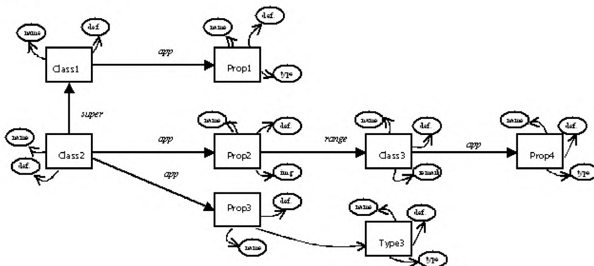
Рисунок Е.1—Определения и взаимоотношения онтологических концепций: экземпляр диаграммы
