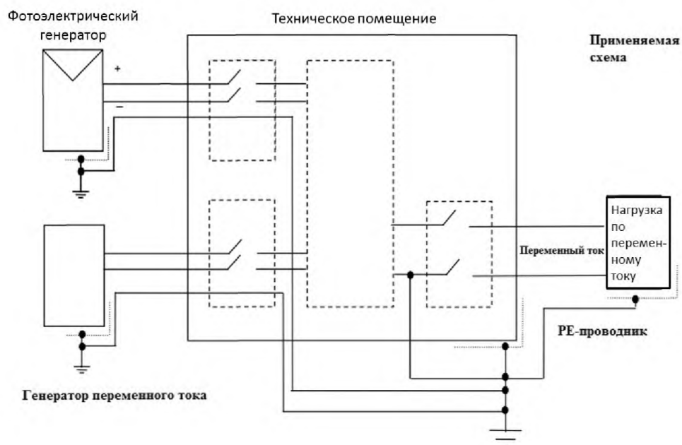
Рисунок 7 — Конфигурации I и K — только солнечная фотозлектрическая батарея индивидуальной или коллективной систем электроснабжения P < 500 \text{ Вт} — с инвертором — d > 15 \text{ м}
