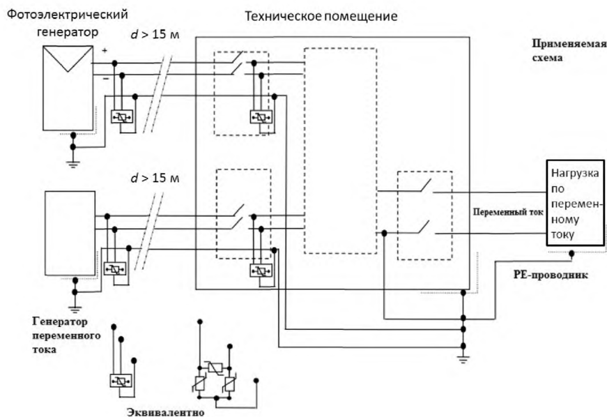
Рисунок 9 — Конфигурация J и L — солнечная фотоэлектрическая батарея совместно с другим генератором индивидуальной или коллективной систем электроснабжения — d > 15 м
