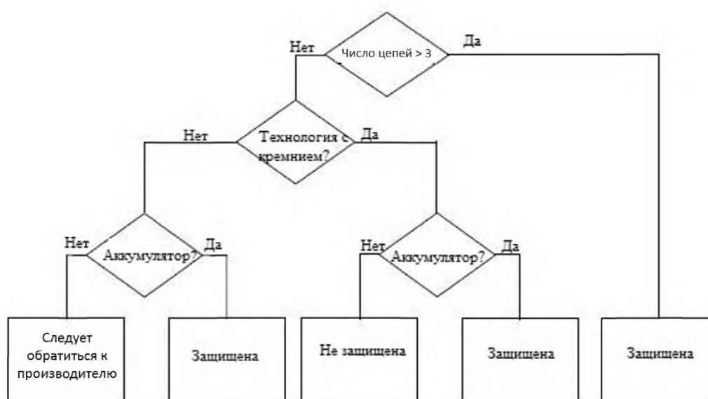
Рисунок 13 — Требования по максимальной токовой защите в фотоэлектрической цепи
