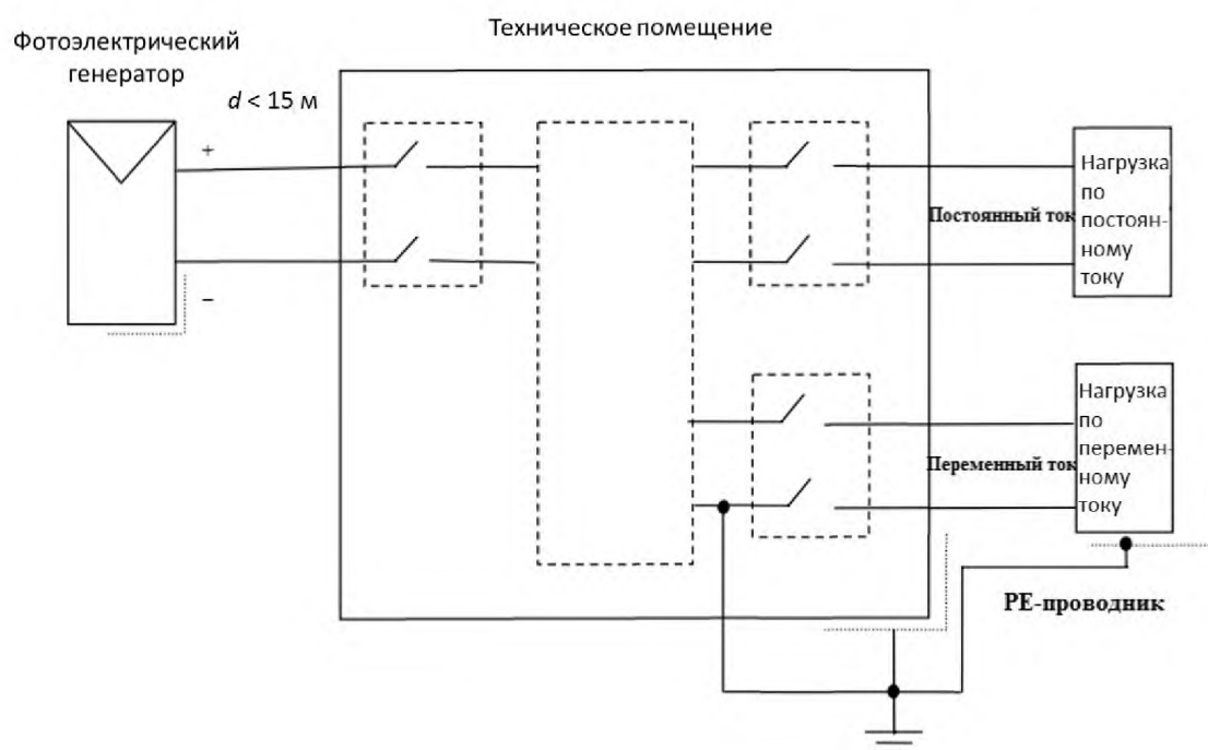
Рисунок 3 — Конфигурация G — только солнечная фотозлектрическая батарея индивидуальной системы электроснабжения P < 500 \text{ Вт} — без инвертора — d > 15 \text{ м}
