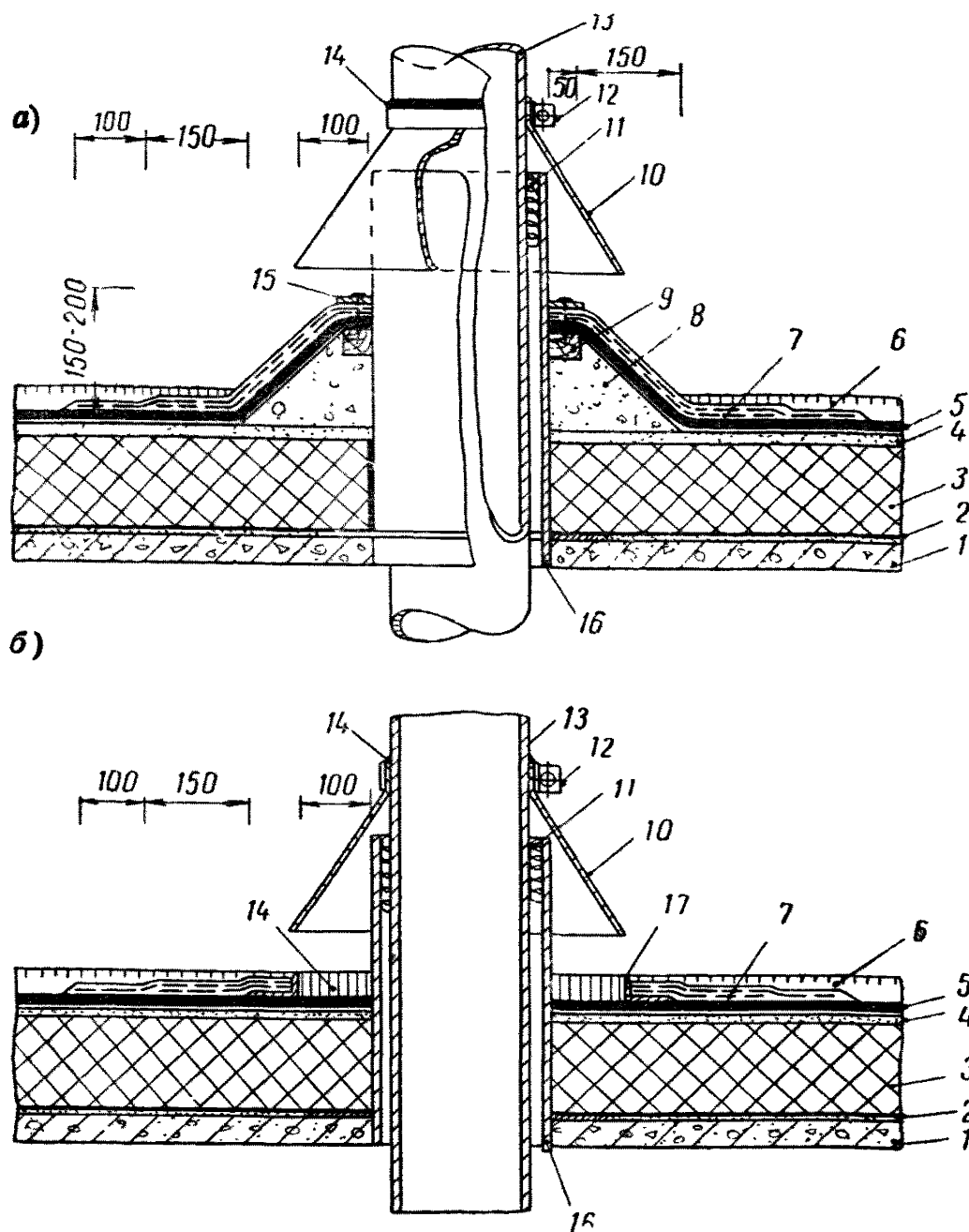
Рис. 6. Примеры решения пропуска труб через мастичную кровлю
