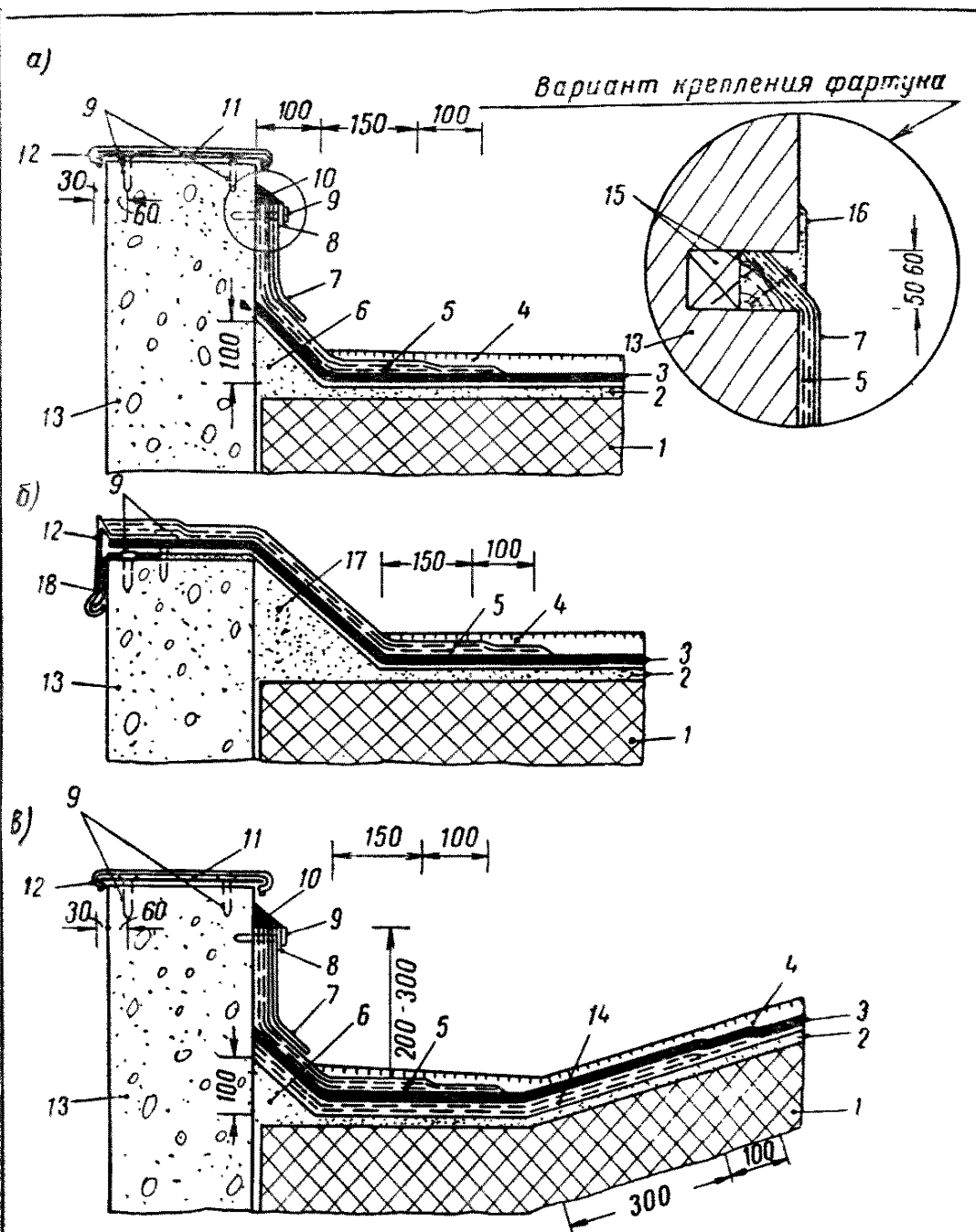
Рис. 2. Примеры решения деталей примыкания мастичной кровли к парапету
