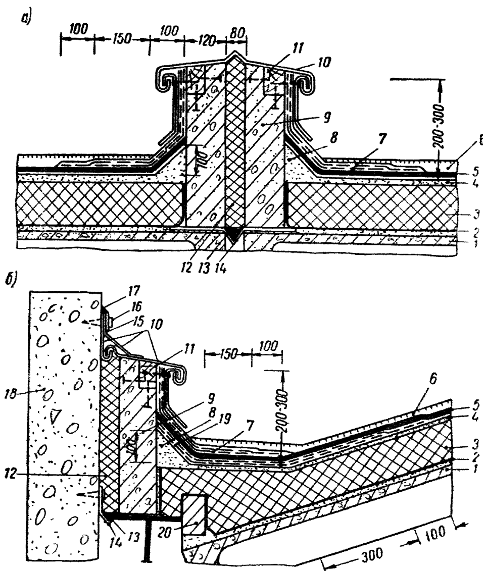
Рис. 3. Детали деформационных швов с вертикальными участками примыкания
