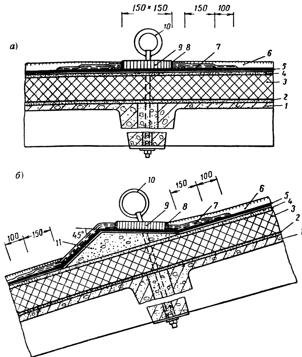
Рис. 7. Примеры решения пропуска анкера через мастичную кровлю
