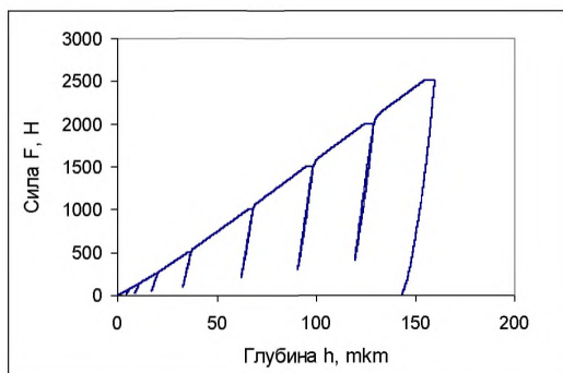
Рисунок 3 – Вид многоциклового диаграммы вдавливания
