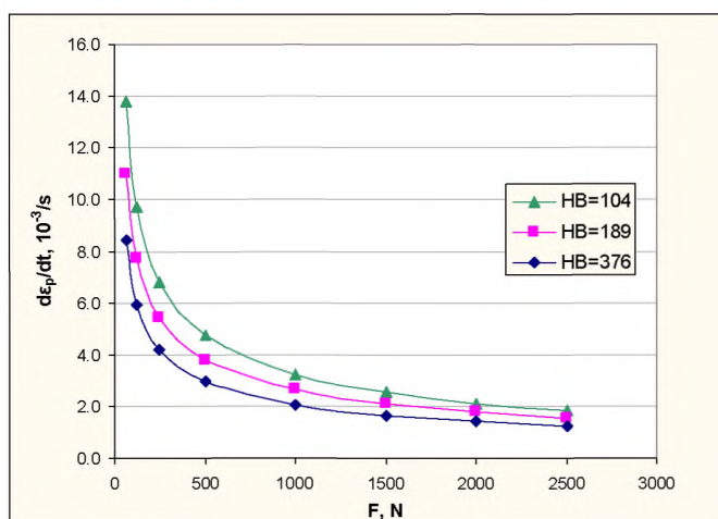
Рисунок В.1 - Изменение скорости эффективной деформации под индентором диаметром 2,5 мм при вдавливании в три образца с различной твердостью при одноцикловом режиме испытания
