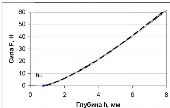
Сплошная линия – участок диаграммы вдавливания, пунктирная линия – линия регрессии; ◦ – найденная точка отсчета
