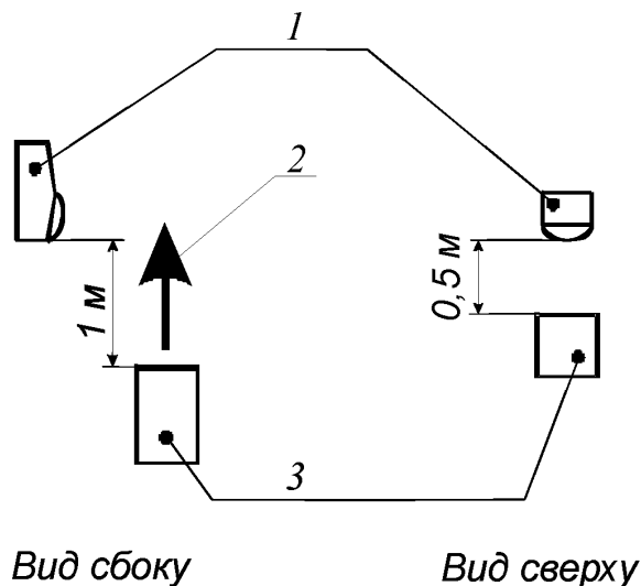
Рисунок 7 — Схема расположения тепловентилятора перед ПОЭИИ
