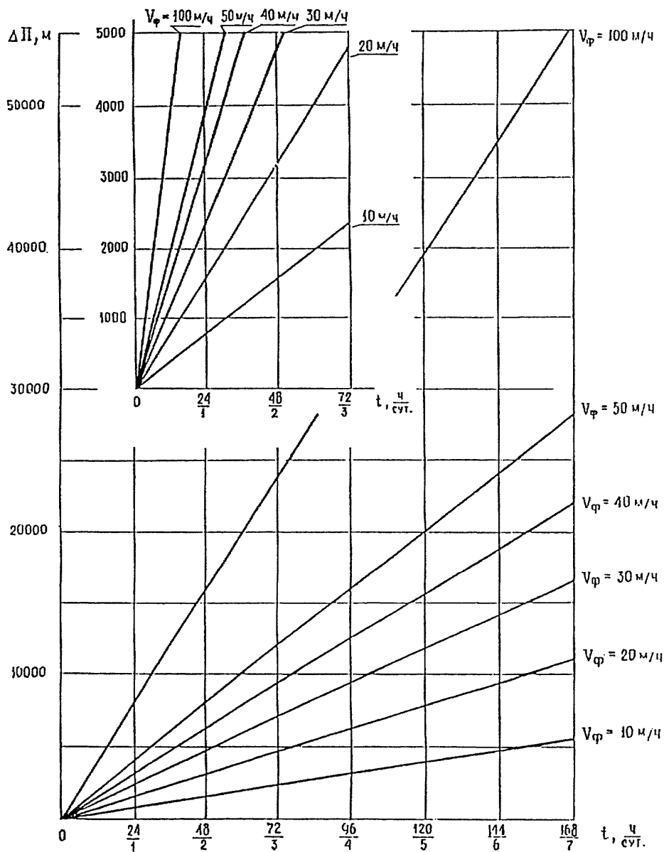
Рис.4.3. Определение приращения периметра \Delta \Pi за время распространения пожара t .
