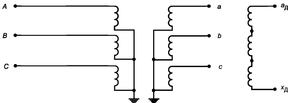
Рисунок Б.3 — Схема включения трехфазных трехобмоточных трансформаторов в трехфазных сетях с изолированной нейтралью и напряжением 3—35 кВ
