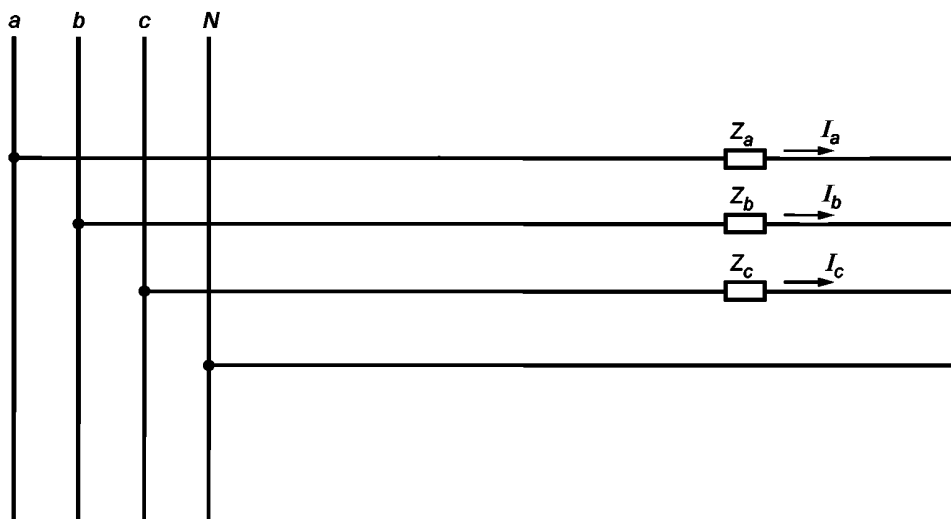
Рисунок Б.7 — Схема соединения нагрузок ТН для четырехпроводной измерительной цепи
