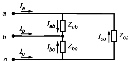
Рисунок Б.6 — Схема соединения нагрузок ТН треугольником для трехпроводной вторичной цепи
