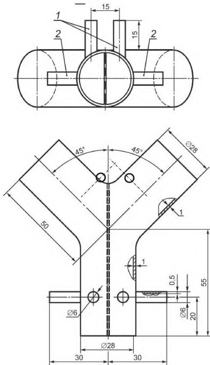
Рисунок А.4 – Тройник для ИДА с загубником
