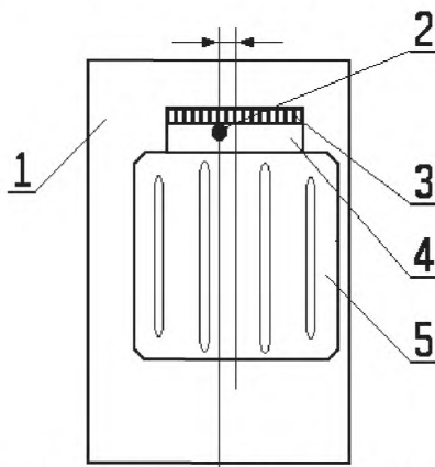
1 – щит; 2 – штырь; 3 – горизонтальная линейка; 4 – приспособление; 5 – ИДА Рисунок 1 – Принципиальная схема стенда для определения смещения центра массы
