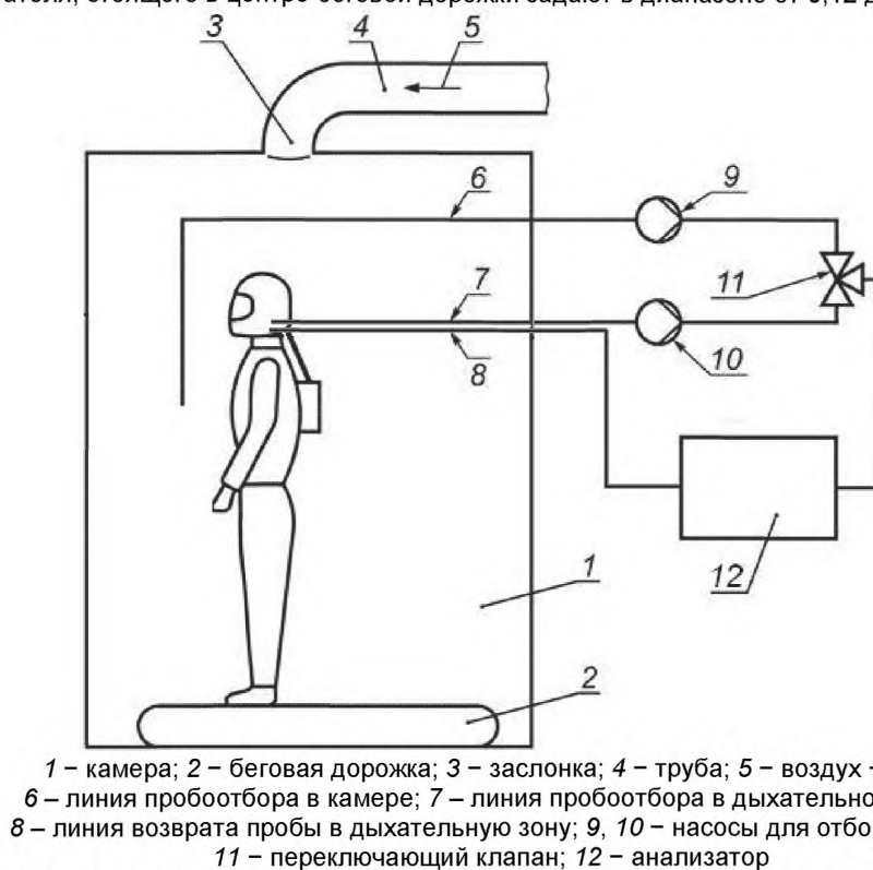
Рисунок 1 – Испытательная установка для определения коэффициента защиты ИДА с использованием гексафторида серы (метод 1)
