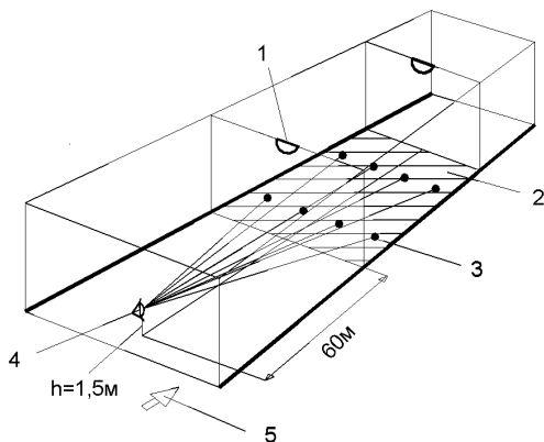
а – схема с фиксированным яркомером
