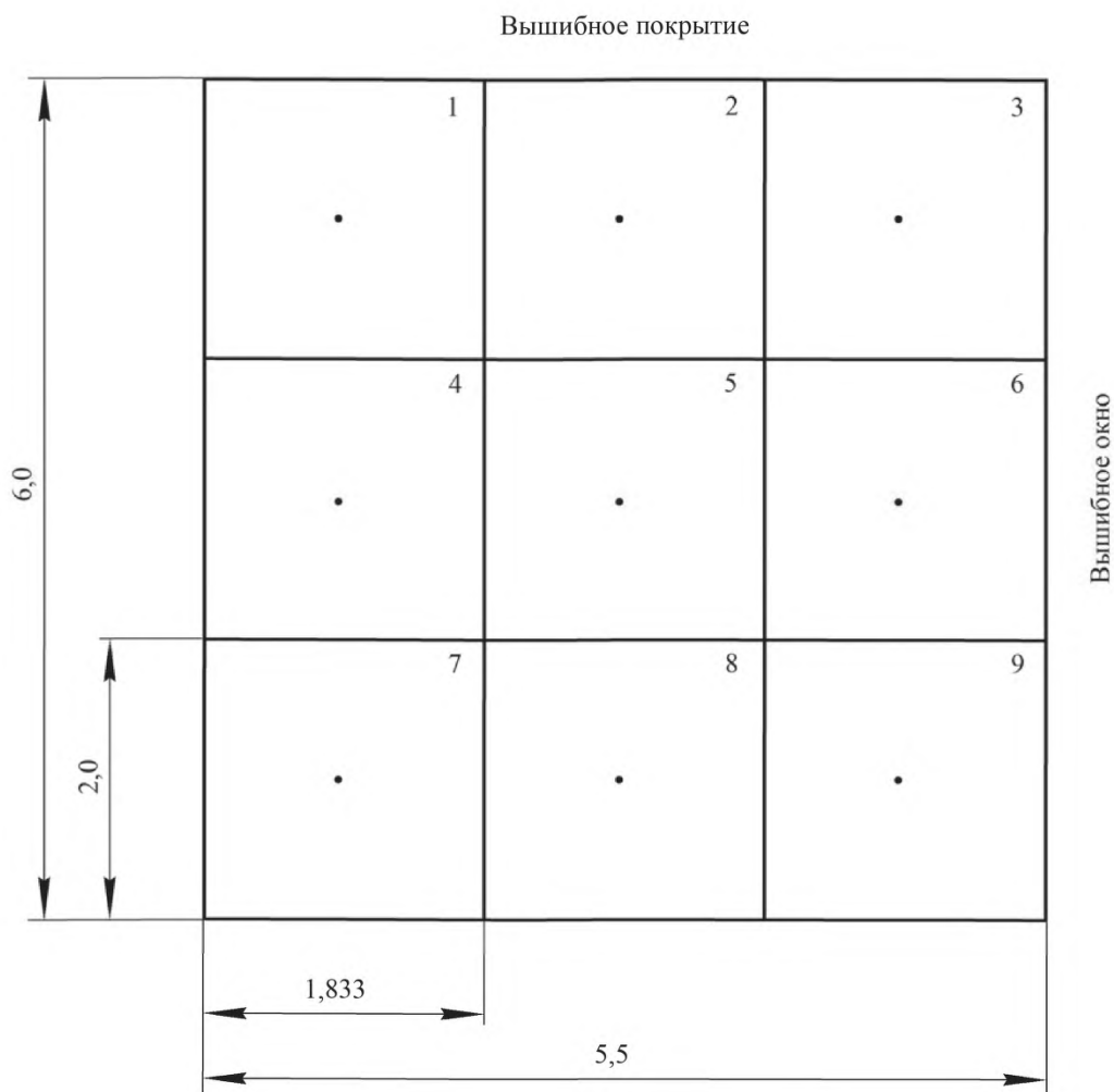
Рисунок А.2 – Схема расположения секторов боковой стены
