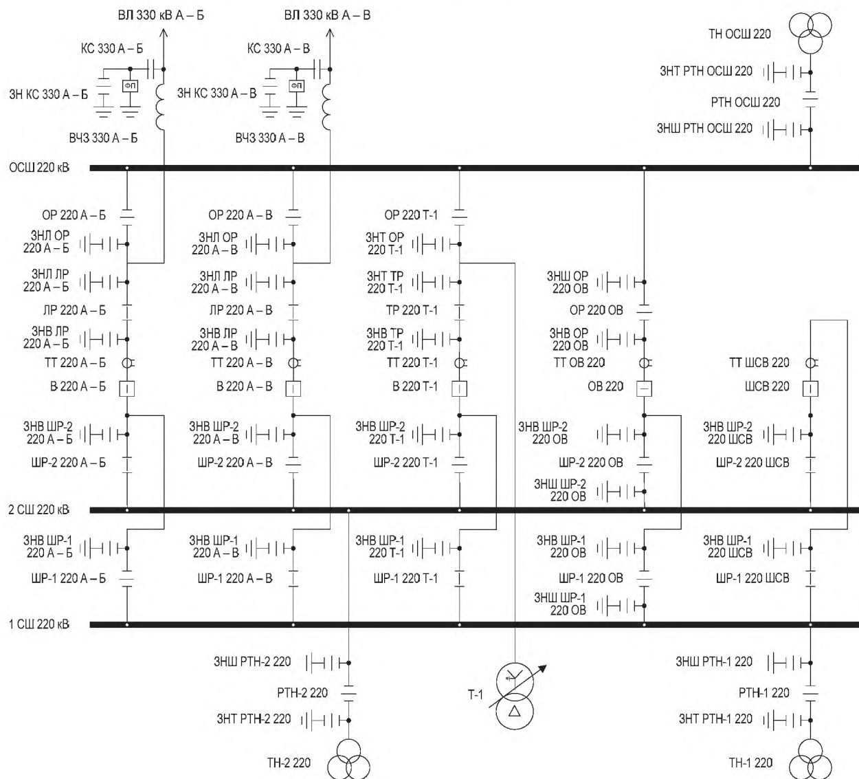
Рисунок Б.1 – Схема РУ 220 кВ типа «две рабочие и обходная системы шин»
