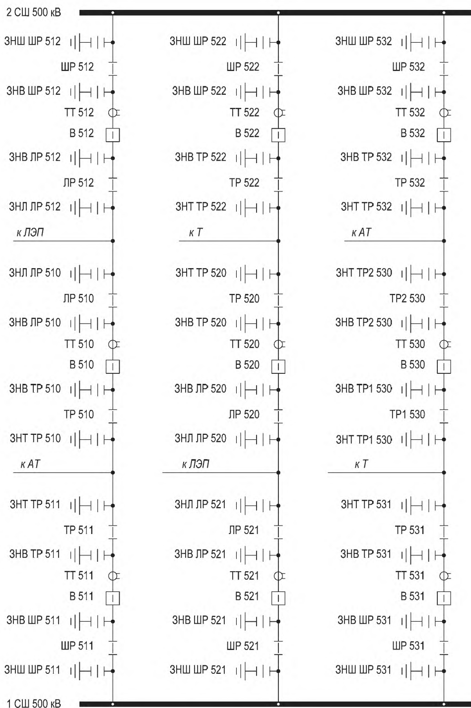
Рисунок Б.4 – Схема РУ 500 кВ типа «трансформаторы – шины с полугорным присоединением линий»
