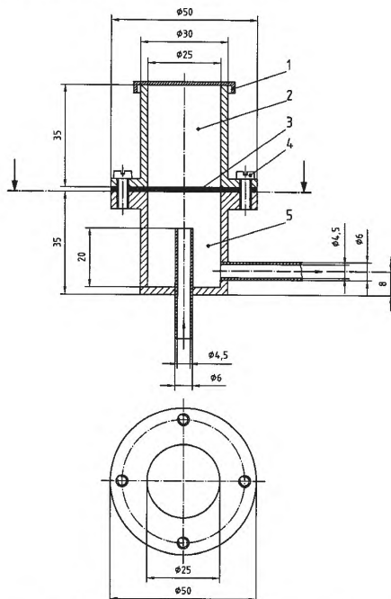
Рисунок 4 — Альтернативная диффузионная ячейка
