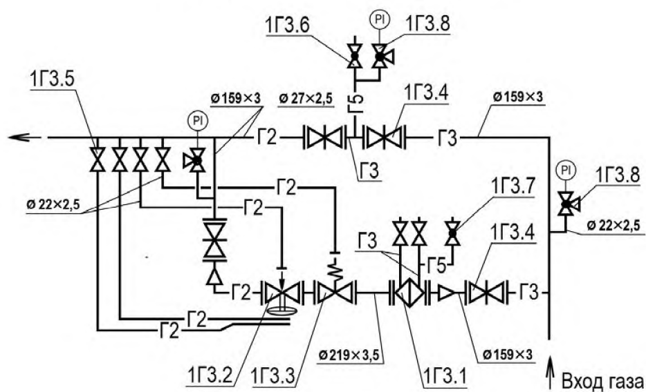
Рисунок Е.1 — Пример выполнения схемы установки
