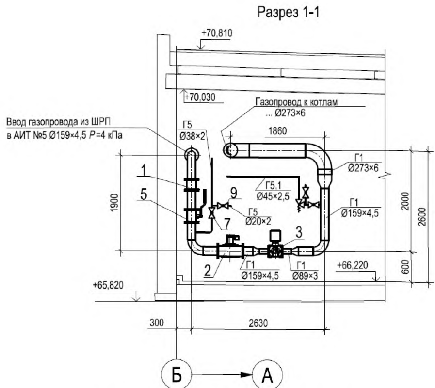
Рисунок В.2 – Пример выполнения разреза для котельной
