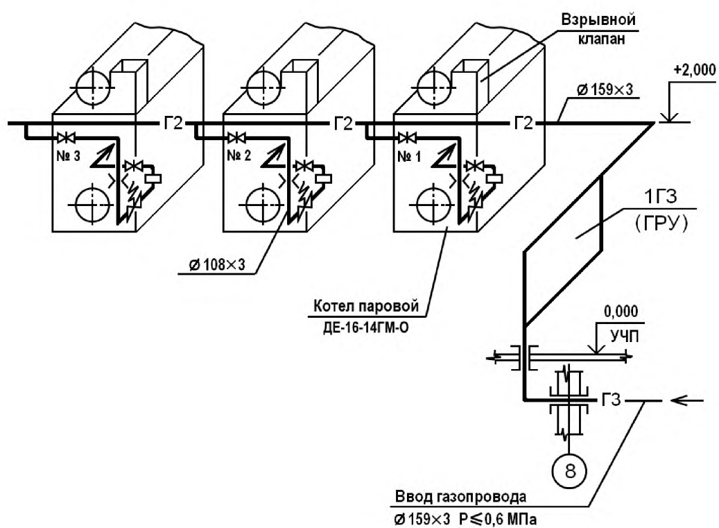
Рисунок Г.1 — Схема газоснабжения котельной
