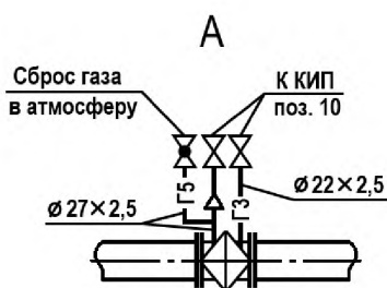
Рисунок Д.3 — Пример выполнения узла
