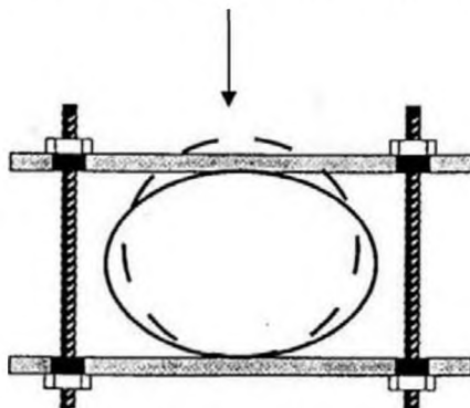
Рисунок В.1 – Схема приложения нагрузки
