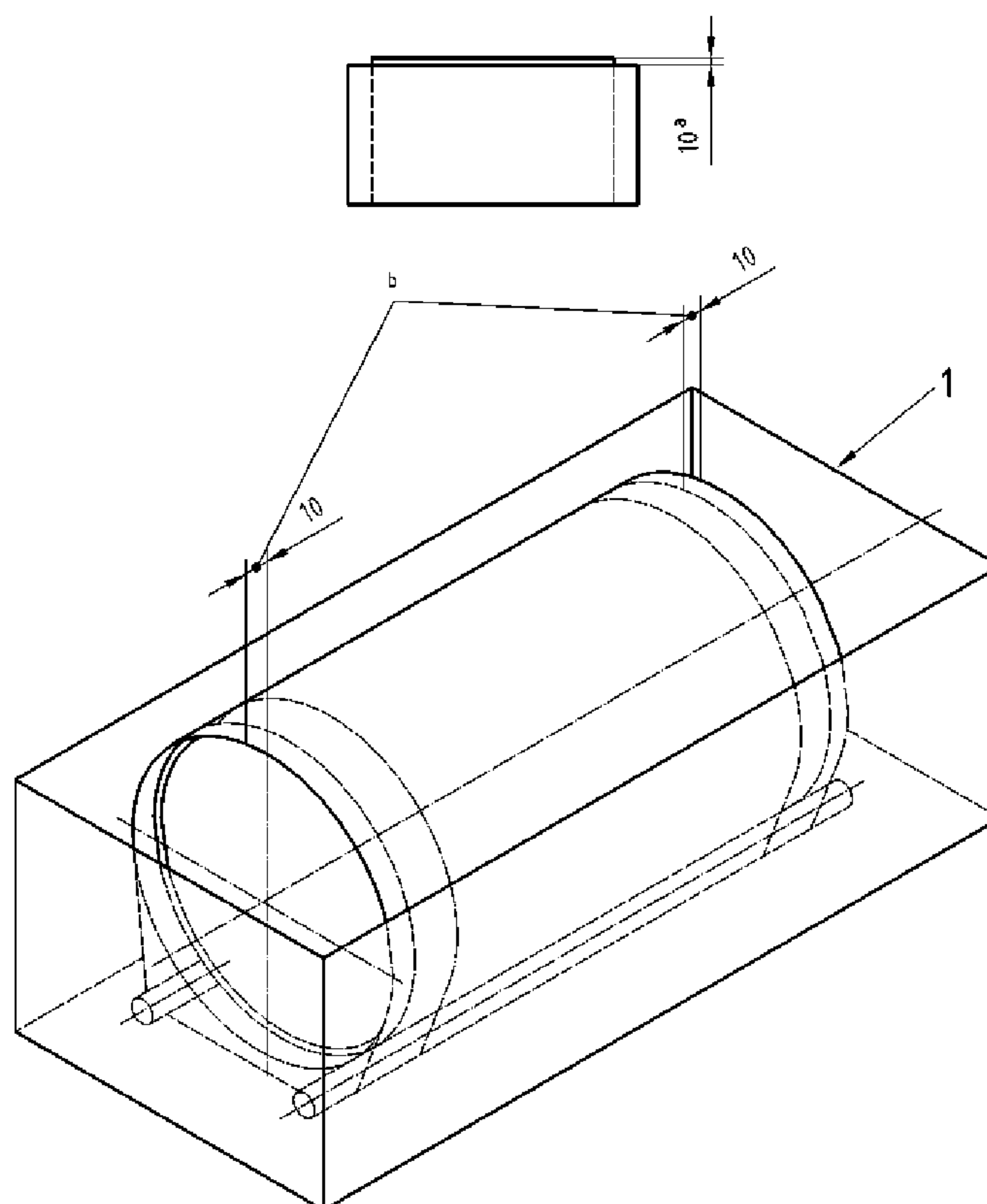
1 — Металлический контейнер
