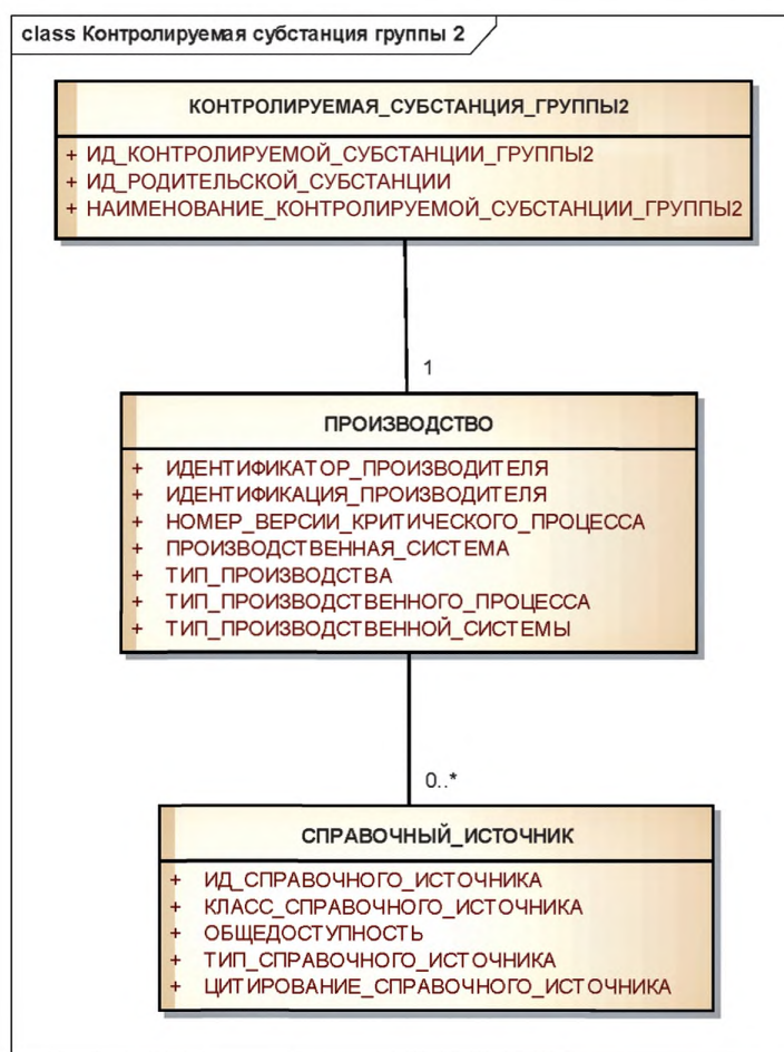
Рисунок 18 — Информационная модель описания контролируемой субстанции группы 2
