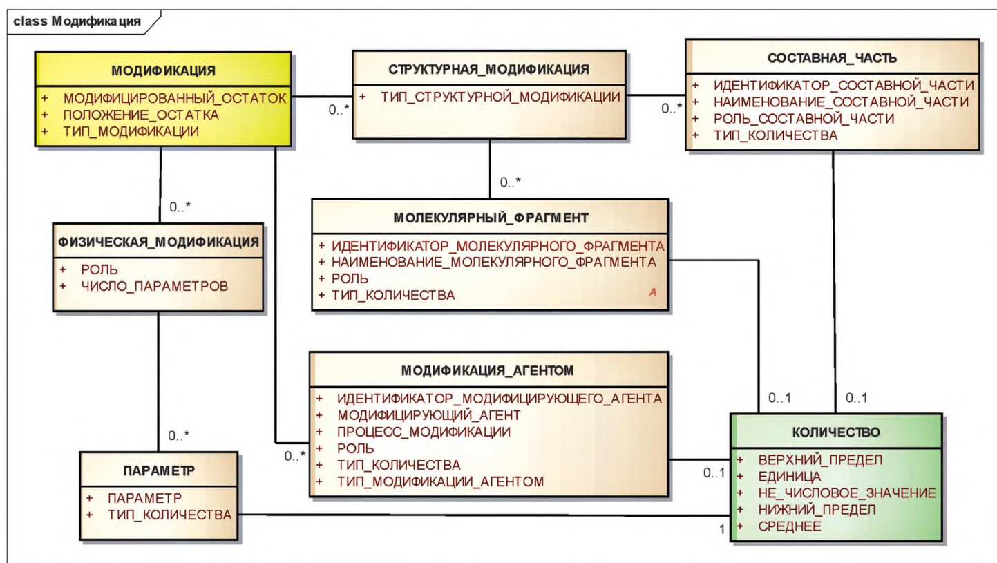
Рисунок 6 — Информационная модель описания модификаций
