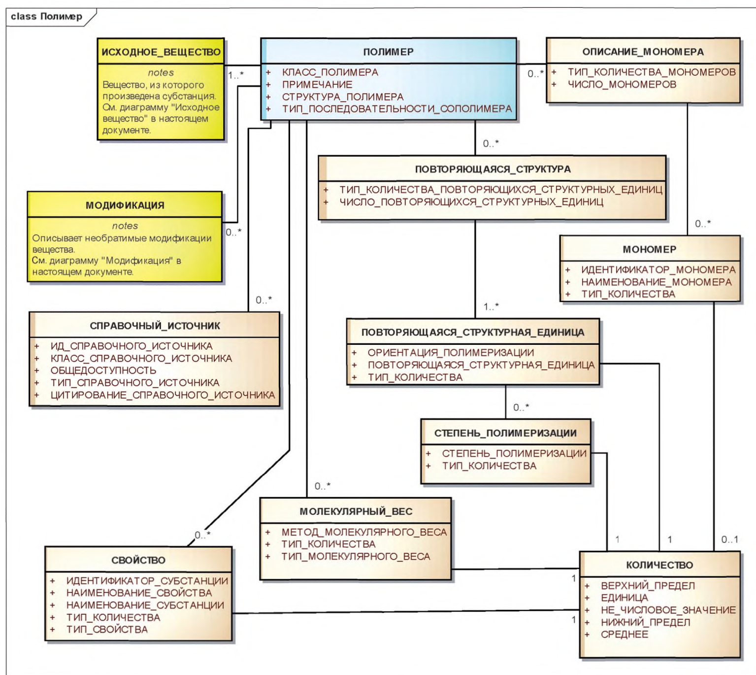
Рисунок 12 — Информационная модель описания полимера
