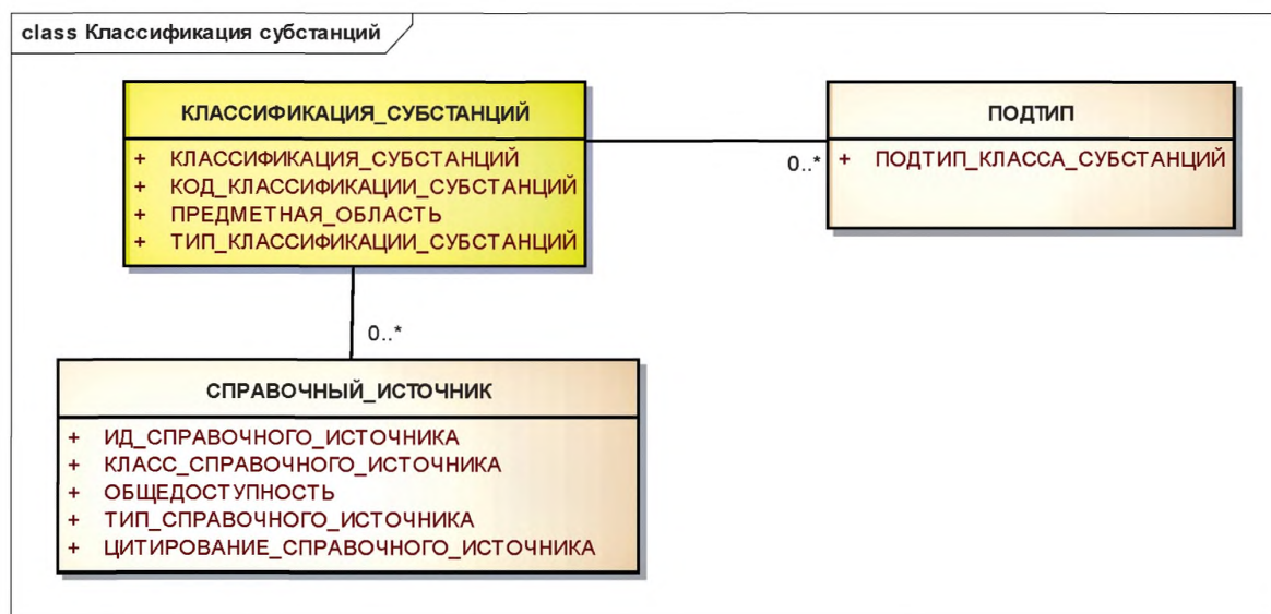
Рисунок 16 — Информационная модель классификации субстанций
