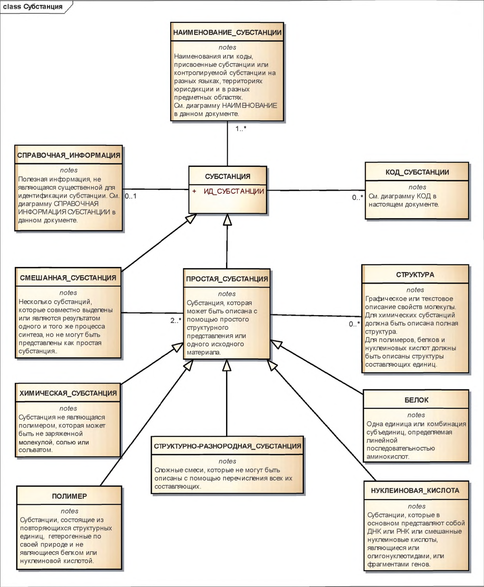
Рисунок 1 — Высокоуровневая информационная модель субстанции
