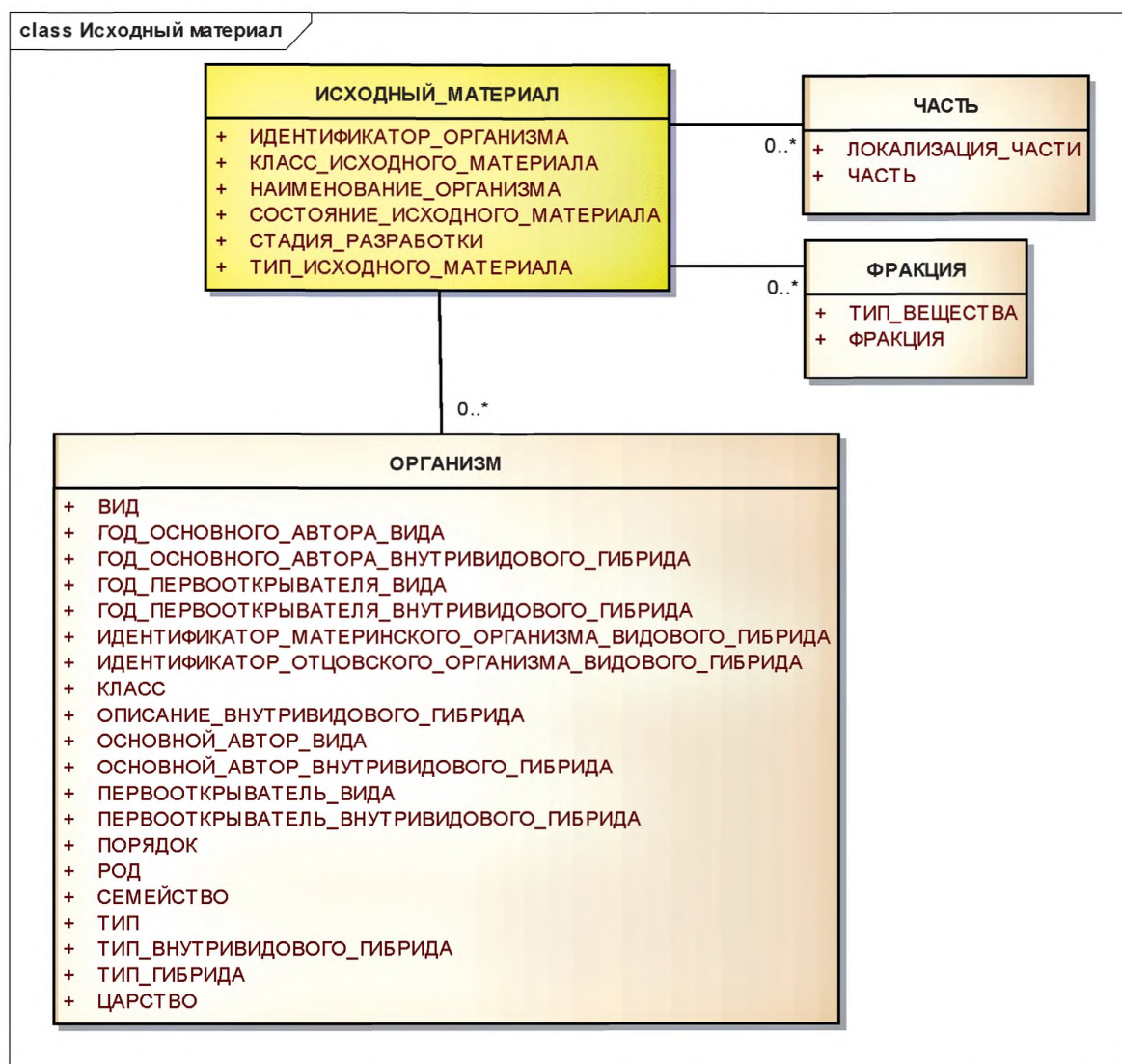
Рисунок 8 — Информационная модель исходного материала
