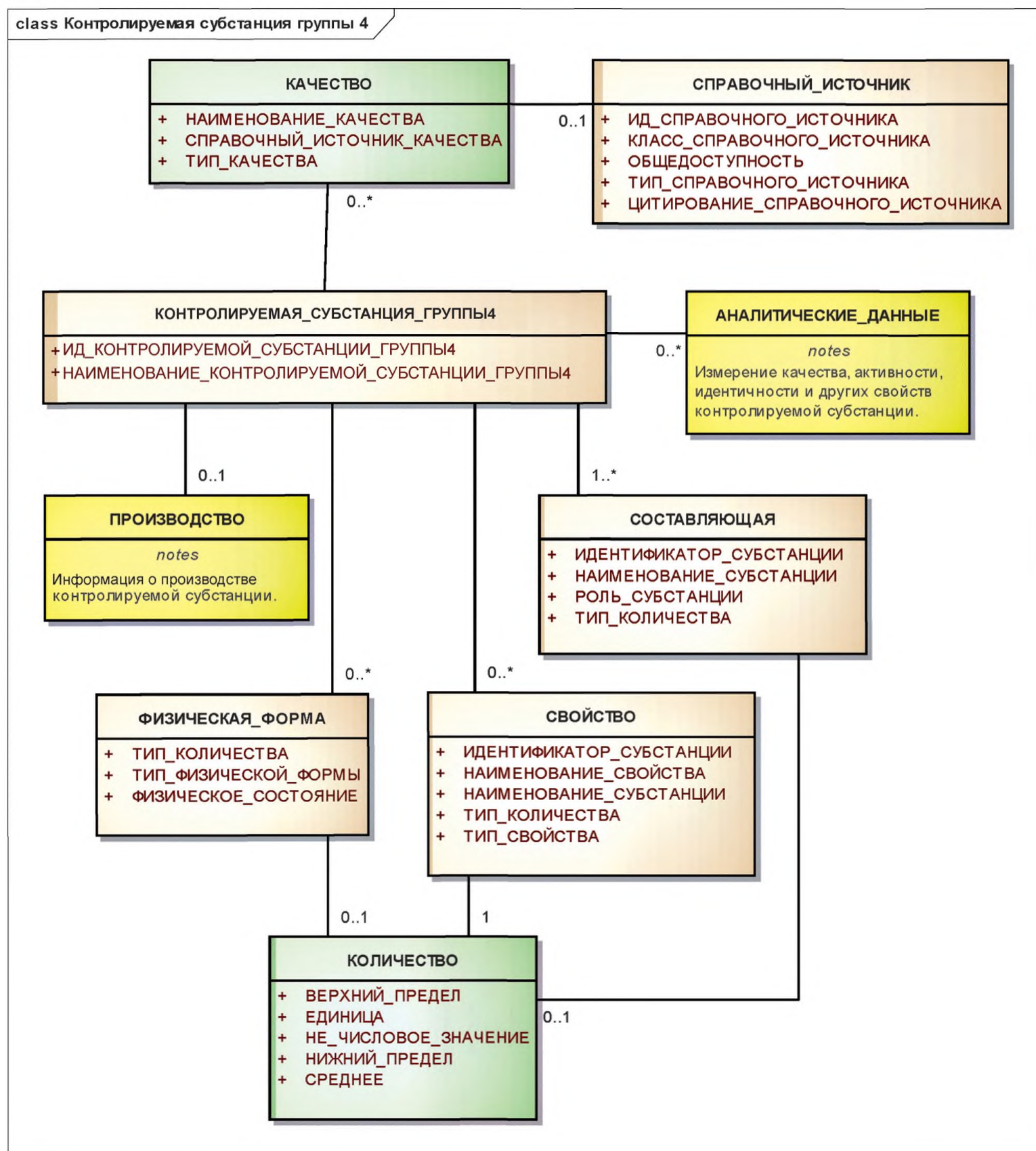
Рисунок 20 — Информационная модель описания контролируемой субстанции группы 4
