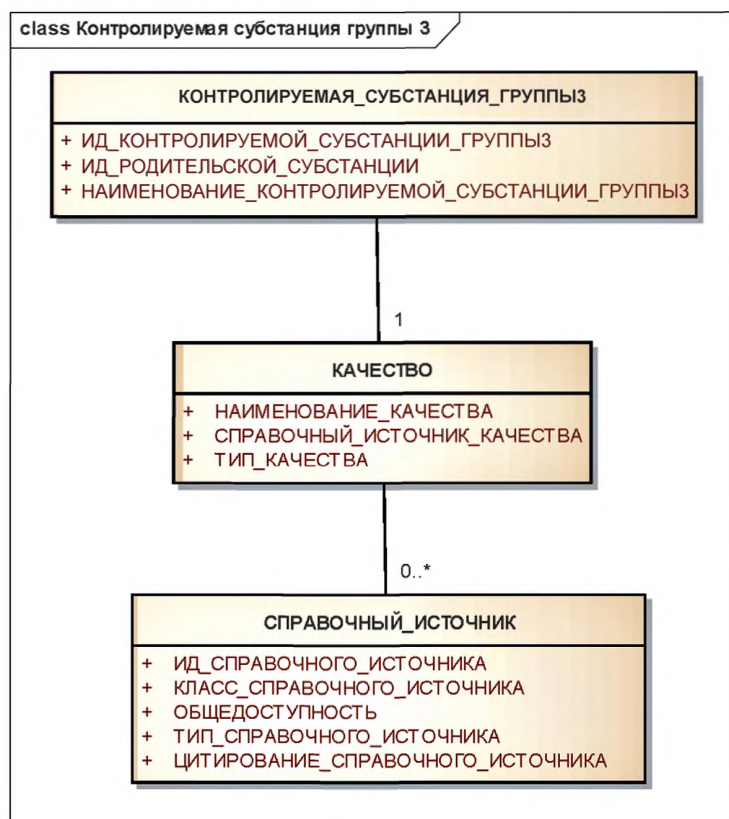
Рисунок 19 — Информационная модель описания контролируемой субстанции группы 3
