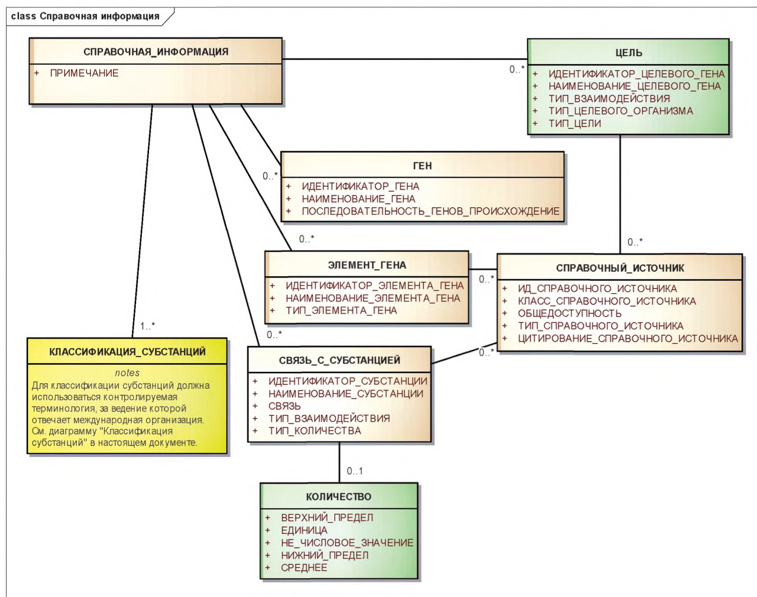
Рисунок 7 — Информационная модель справочной информации
