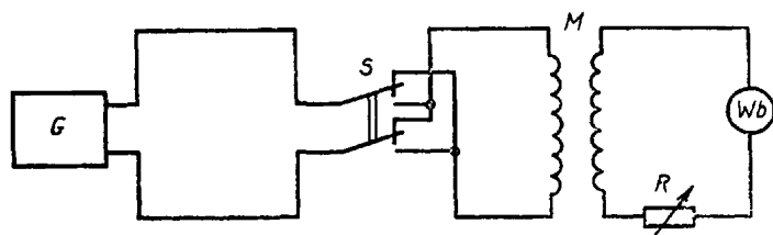
G —калибратор тока; S —переключатель; M —образцовая катушка магнитного потока 1-го разряда; R —магазин сопротивлений; Wb —веряемый веберметр
