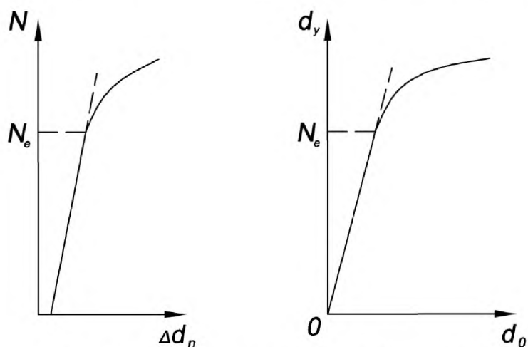
Рисунок А.2.1 — Диаграмма зависимости деформаций
