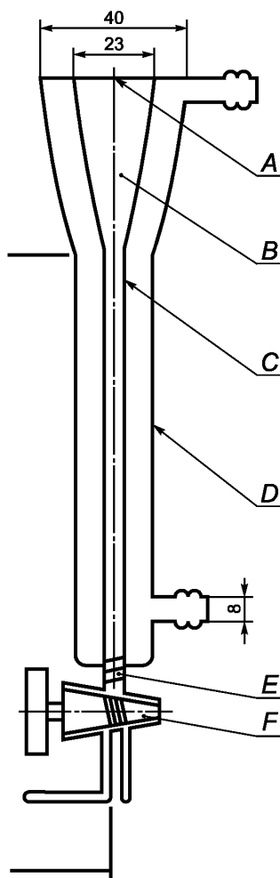
A — место соединения с муфтой из матового стекла; B — свободное пространство; C — внутренняя часть колонки; D — внешняя часть колонки; E — пробка из стекловолкна; F — запорный кран
