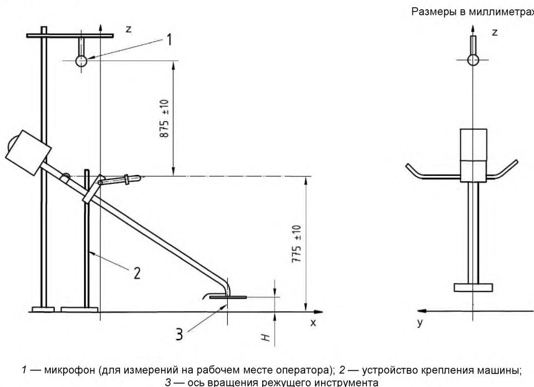
Рисунок В.1 — Испытательная установка для мотокос и кусторезов с встроенным двигателем и точкой подвеса
