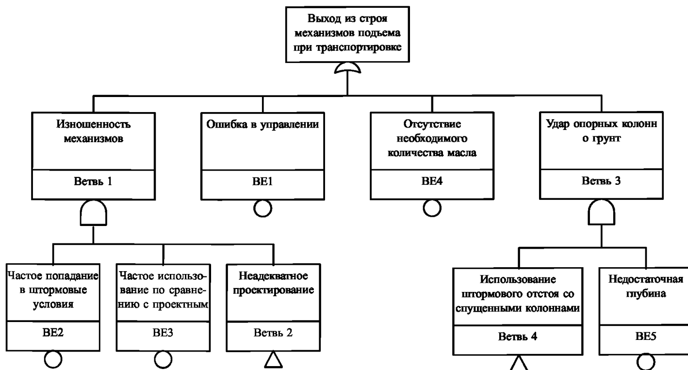
Начальное построение дерева ошибок и неполадок
