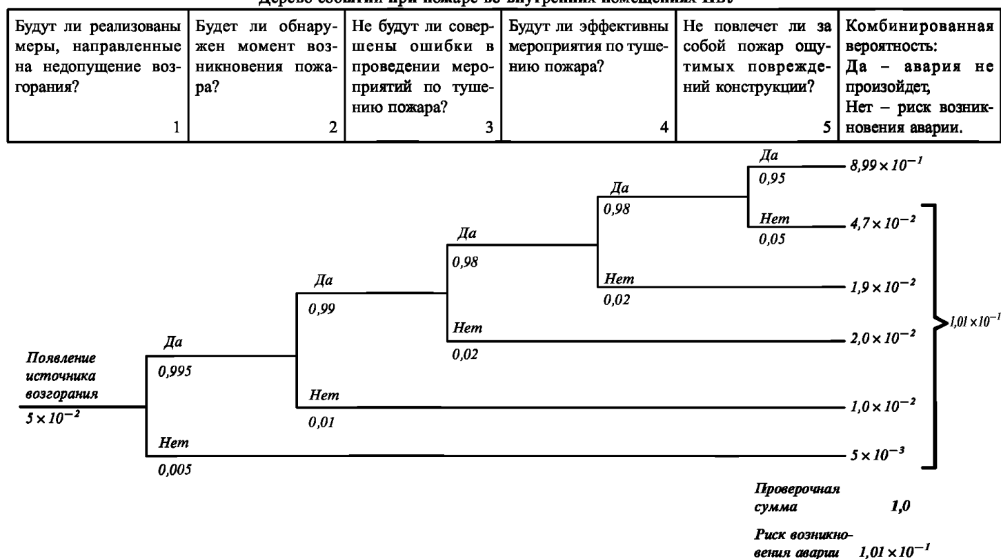
Дерево событий при пожаре во внутренних помещениях ПБУ
