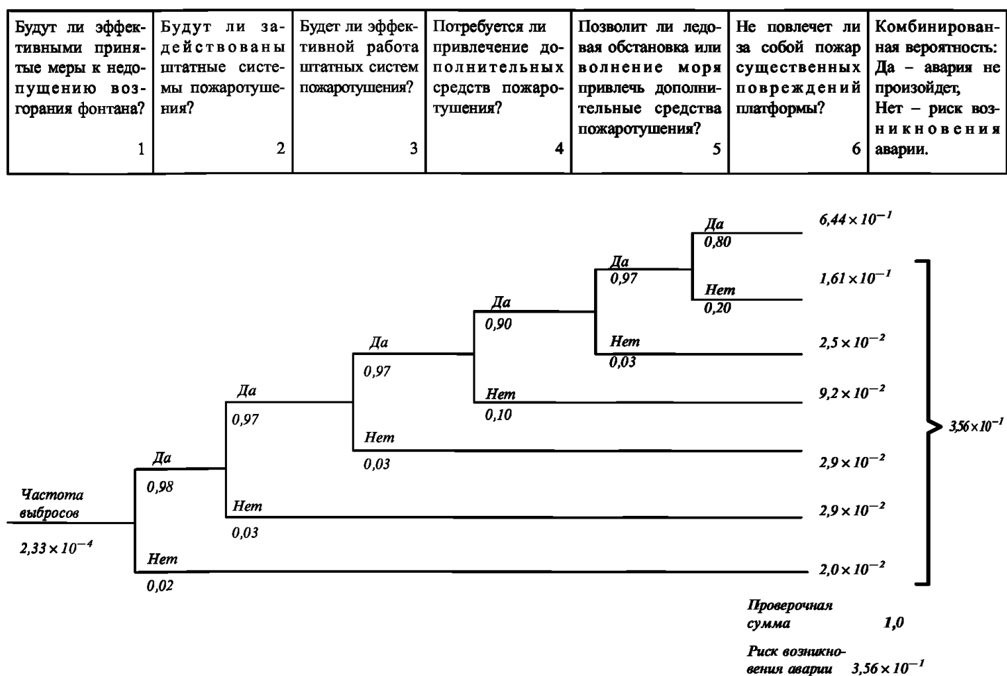
Дерево событий при пожаре фонтана на платформе
