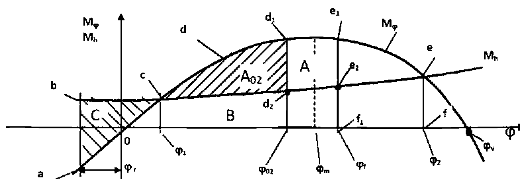
Рис. 3.1.1-1 Диаграмма статической остойчивости с учетом качки:
