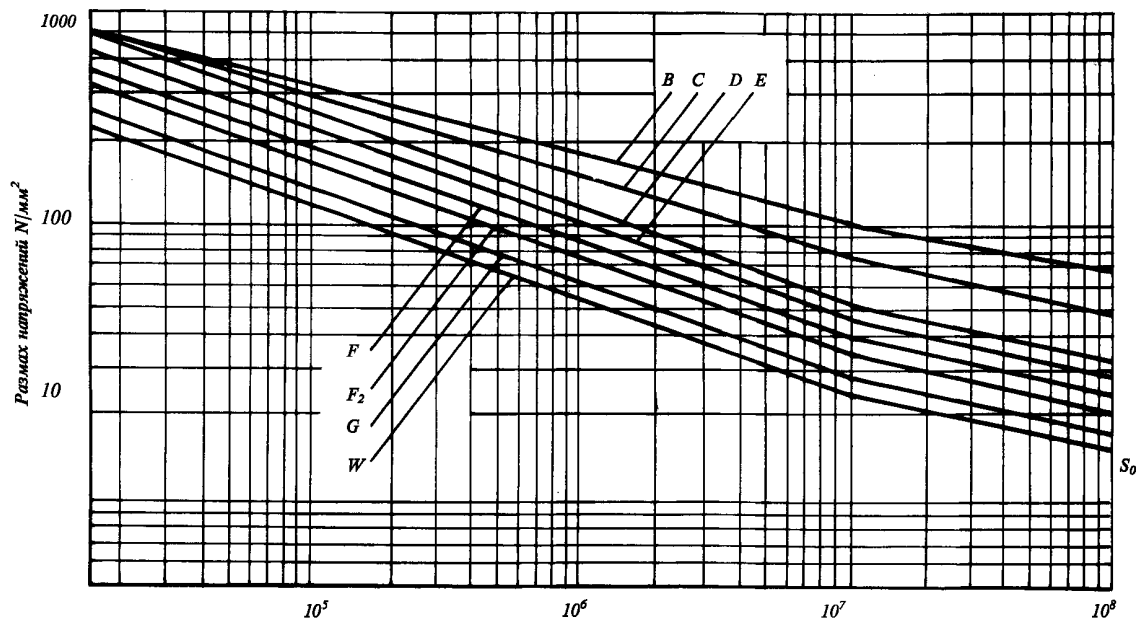
Рис. 2.4.4.8-1 Кривые усталости
