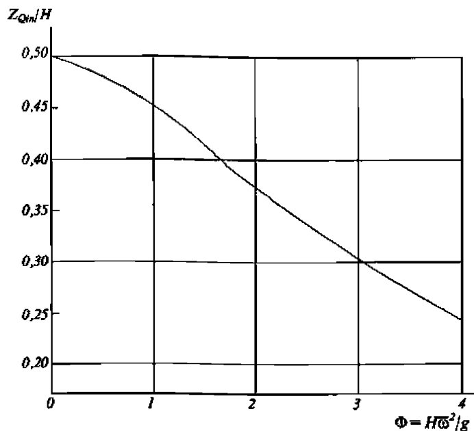
Рис. 3.1.4.13-3 Зависимость Z_{Qin}/H от параметра \Phi = H\bar{\omega}^2/g
