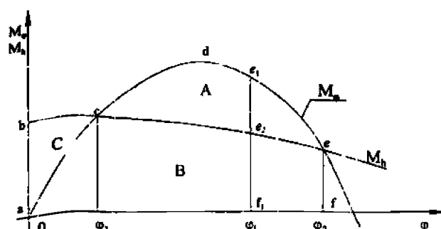
Рис. 3.1.1-2 Диаграмма статической остойчивости без учета качки
