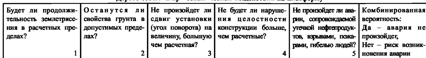
Дерево событий при сейсмическом воздействии на платформу
