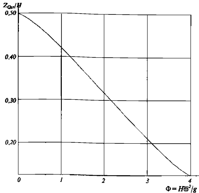
Рис. 3.1.4.13-2 Зависимость Z_{Qsr}/H от параметра \Phi = H\bar{\omega}^2/g
