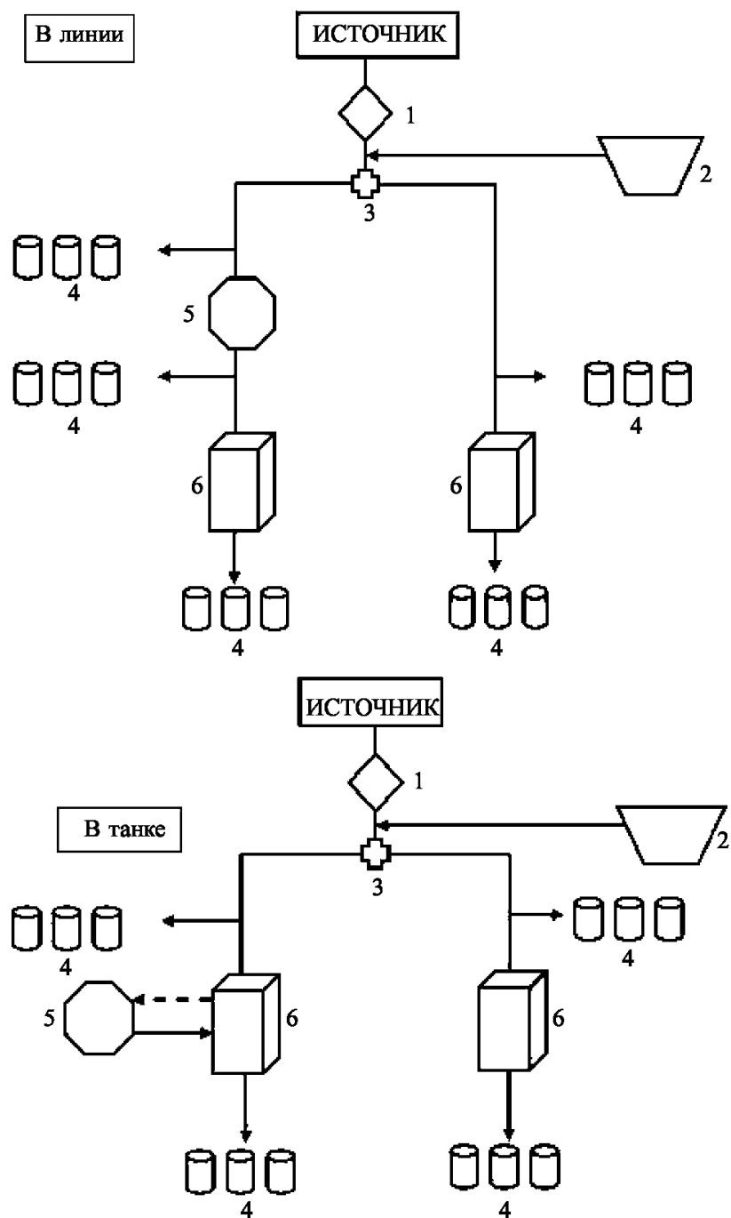
Рис. 3.2 Схематическое устройство возможных испытательных установок для проведения испытаний на стенде
