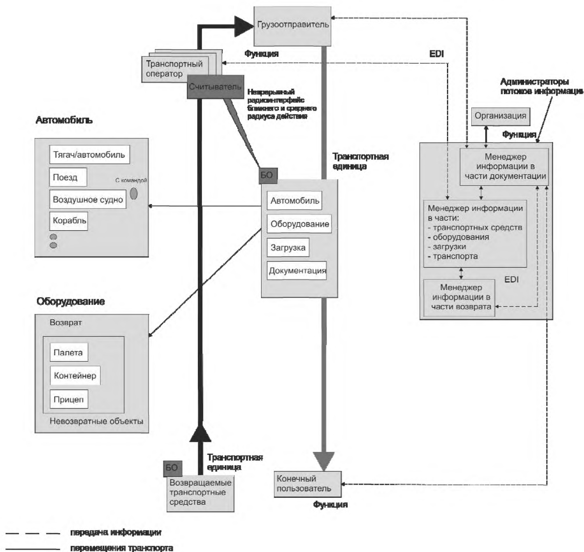
Рисунок 2 — Концептуальный вид системы AVI/AEI
