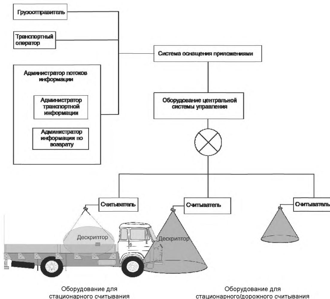
Рисунок 7с — Физическая архитектура
