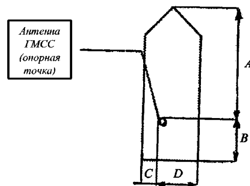
Рис. 5.3 Параметры расположения антенны:
