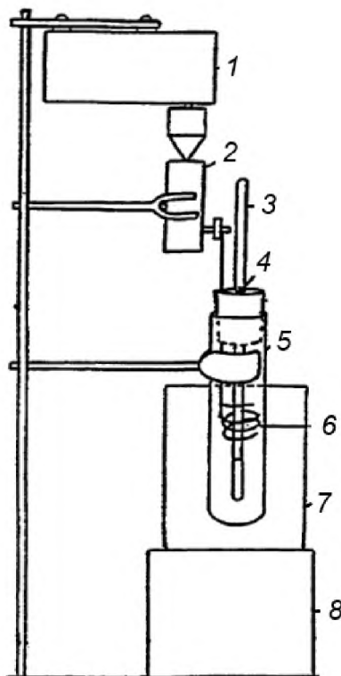
1 – вращающий электродвигатель; 2 – преобразователь вращательного движения в поршневое; 3 – термистор; 4 – корковая пробка; 5 – контейнер для образца (пробирка); 6 – проволоочная мешалка в верхнем положении; 7 – баня; 8 – подставка для бани
