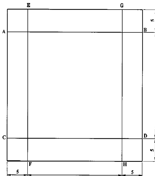
Рисунок 1 – Маркировка образца для испытаний
