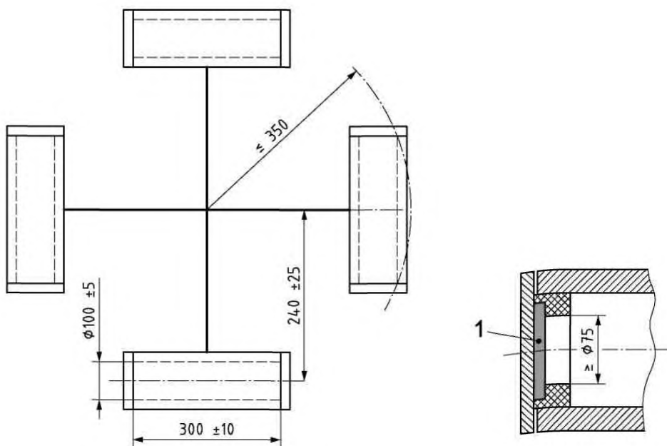
Рисунок 1 — Графическая схема (не в масштабе) загрязняющей барабанной машины, отвечающей необходимым требованиям
