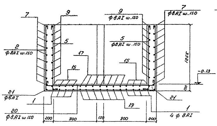
Сечение 5-5
