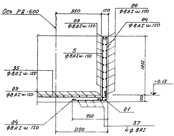
Сечение 7-7
