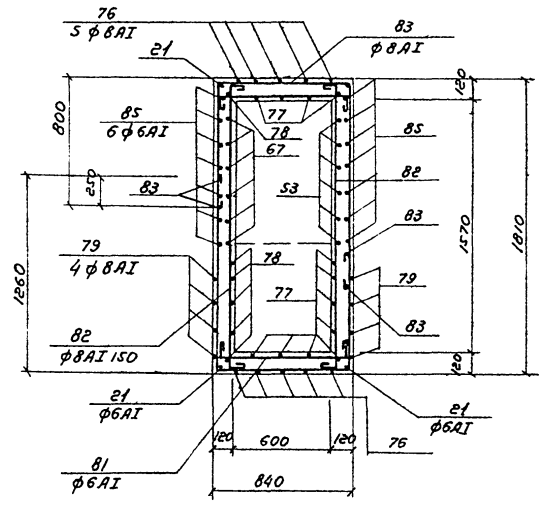
Сечение 8-8
