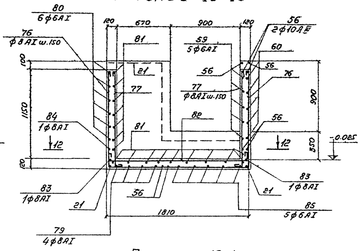
Плн по 12-12
