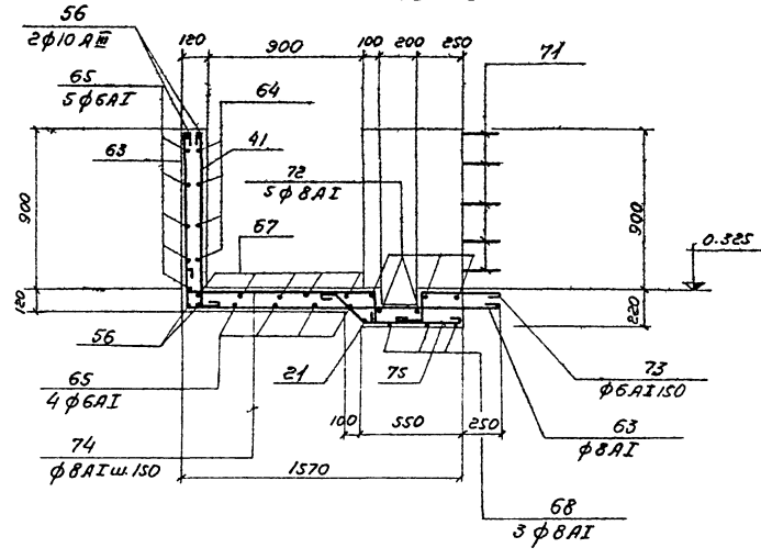
Сечение 9-9
