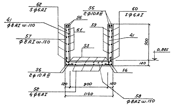
Сечение 9-9
