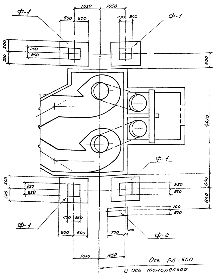
Монтажный план фундаментов
