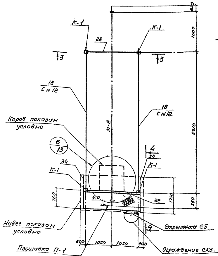
Монтажная схема монорейса
