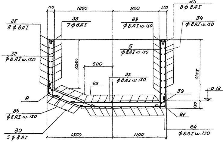
Сечение 7-7
