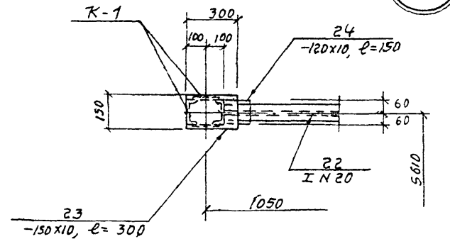
№ 3-3 (см лист КЖ-20)
