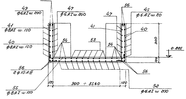
Сечение 8-8
