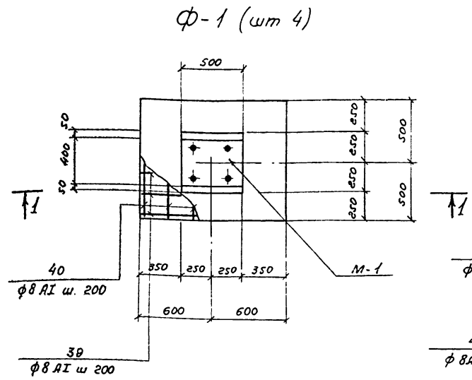
Монтажный план фундаментов
