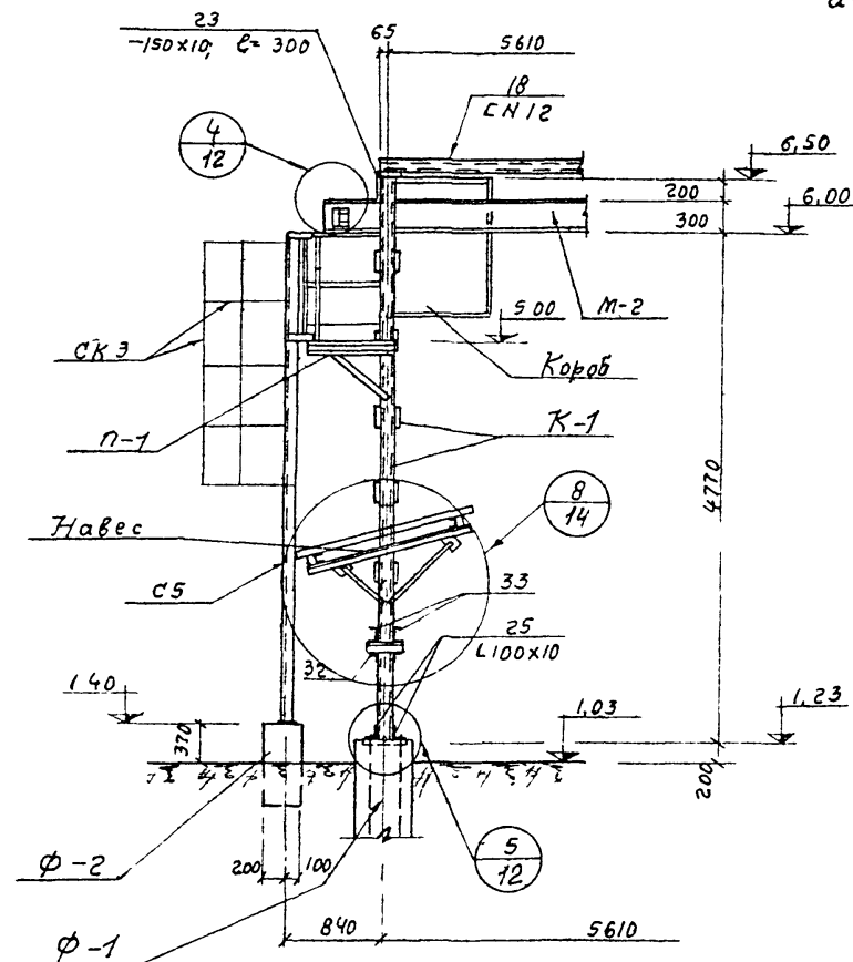
№ 4-4 (см. лист КЖ-20)
