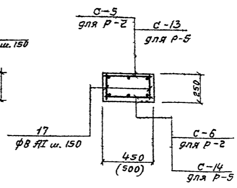
Сечение 5-5
