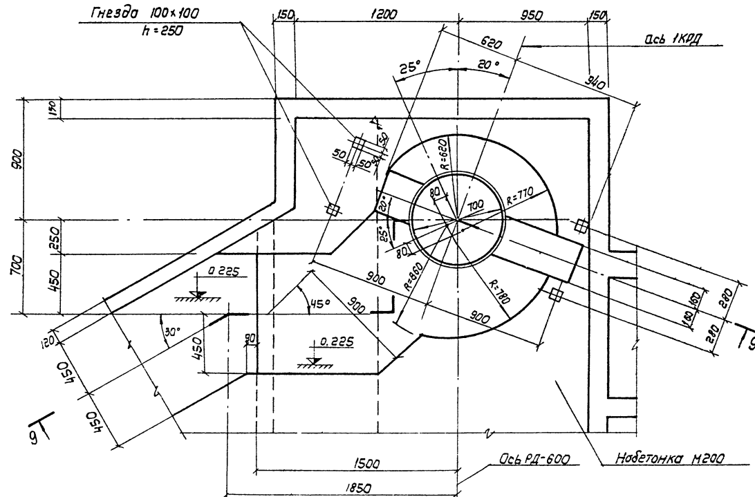
Элемент плана "1" для установки 1КРД
