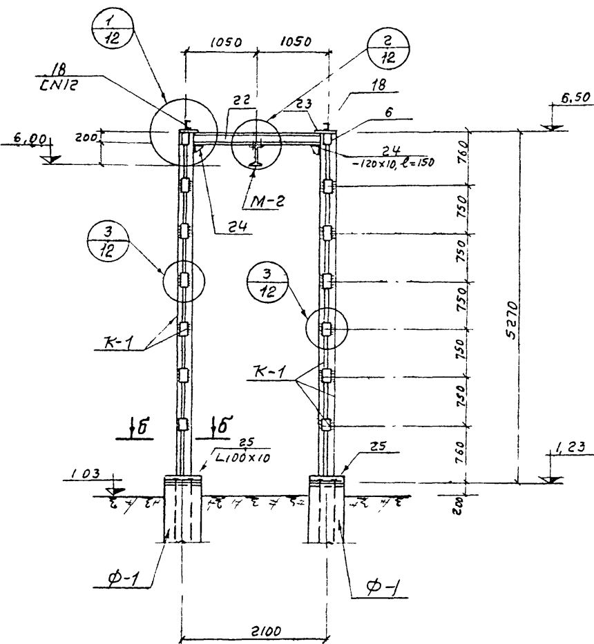
№ 3-3 (см лист КЖ-20)
