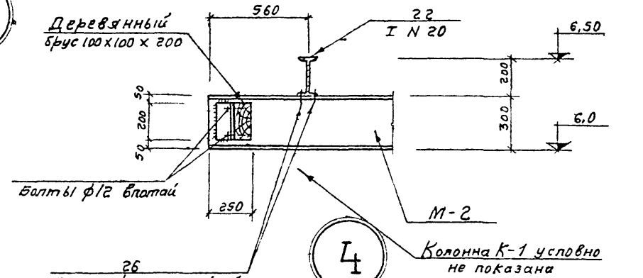
№ 4-4 (см. лист КЖ-20)
