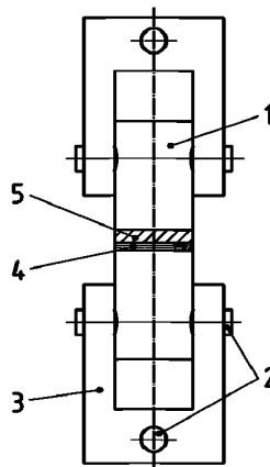
Рисунок 1 – Иллюстрация нагрузочного блока, позволяющего минимизировать внеосевую нагрузку
