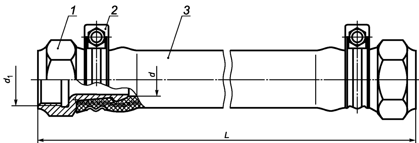
1 — наконечник; 2 — хомут; 3 — рукав по ГОСТ 1335
