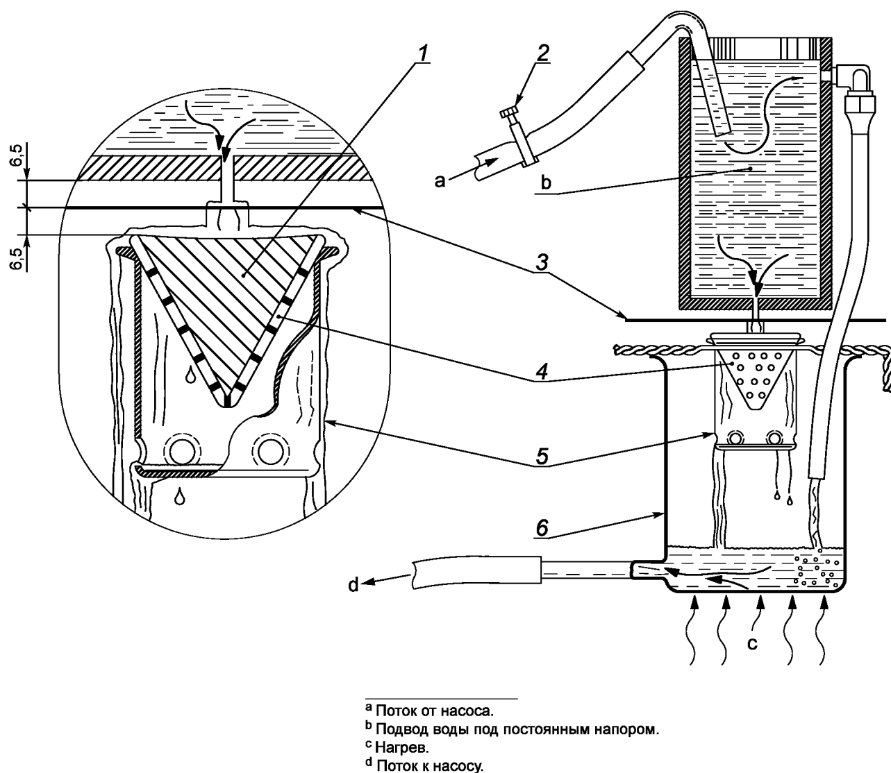
1 — проба смазки в фильтрующем конусе; 2 — регулирующий поток клапан; 3 — медная экранирующая сетка с ячейками размером 1,6 мм; 4 — фарфоровый конус диаметром 50 мм; 5 — лабораторный стакан вместимостью 100 мл с отверстиями; 6 — лабораторный стакан вместимостью 1000 мл с боковым патрубком
