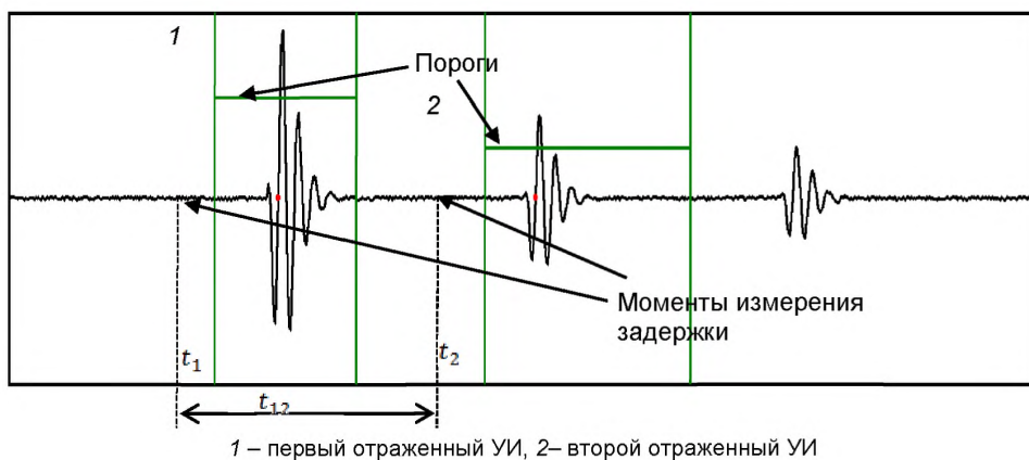
Рисунок 1 – Осциллограмма УИ
