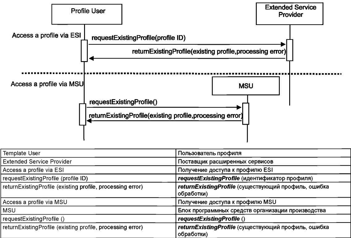
Рисунок 9 — Служба accessProfile
