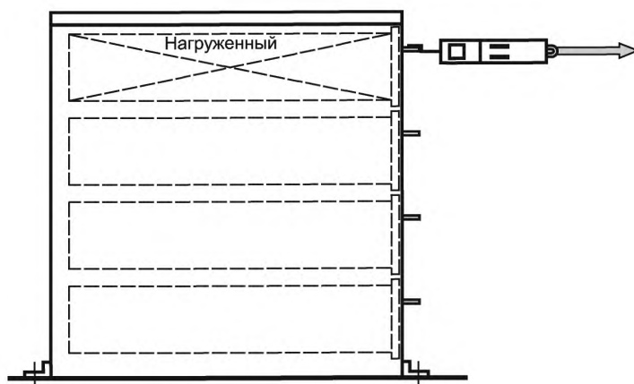
Рисунок 7 — Испытание на тянущее усилие
