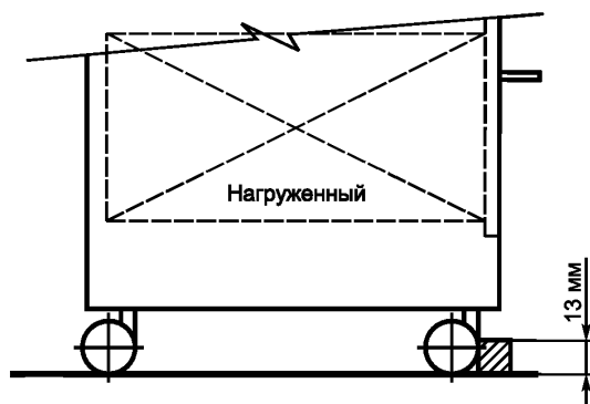
Рисунок 1 — Установка картотек для проведения испытаний
