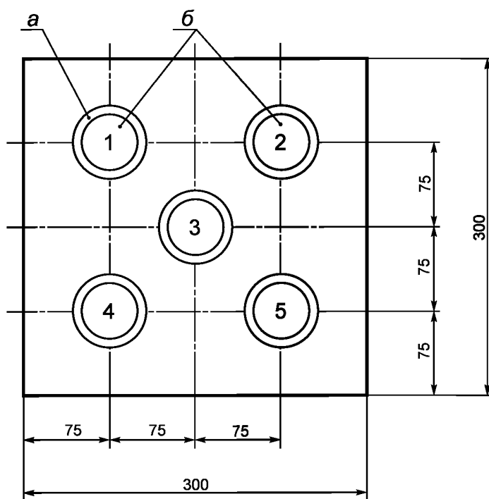
а — цилиндрический пропил; б — образец-кern; 1—5 — маркировка образцов-кернов
