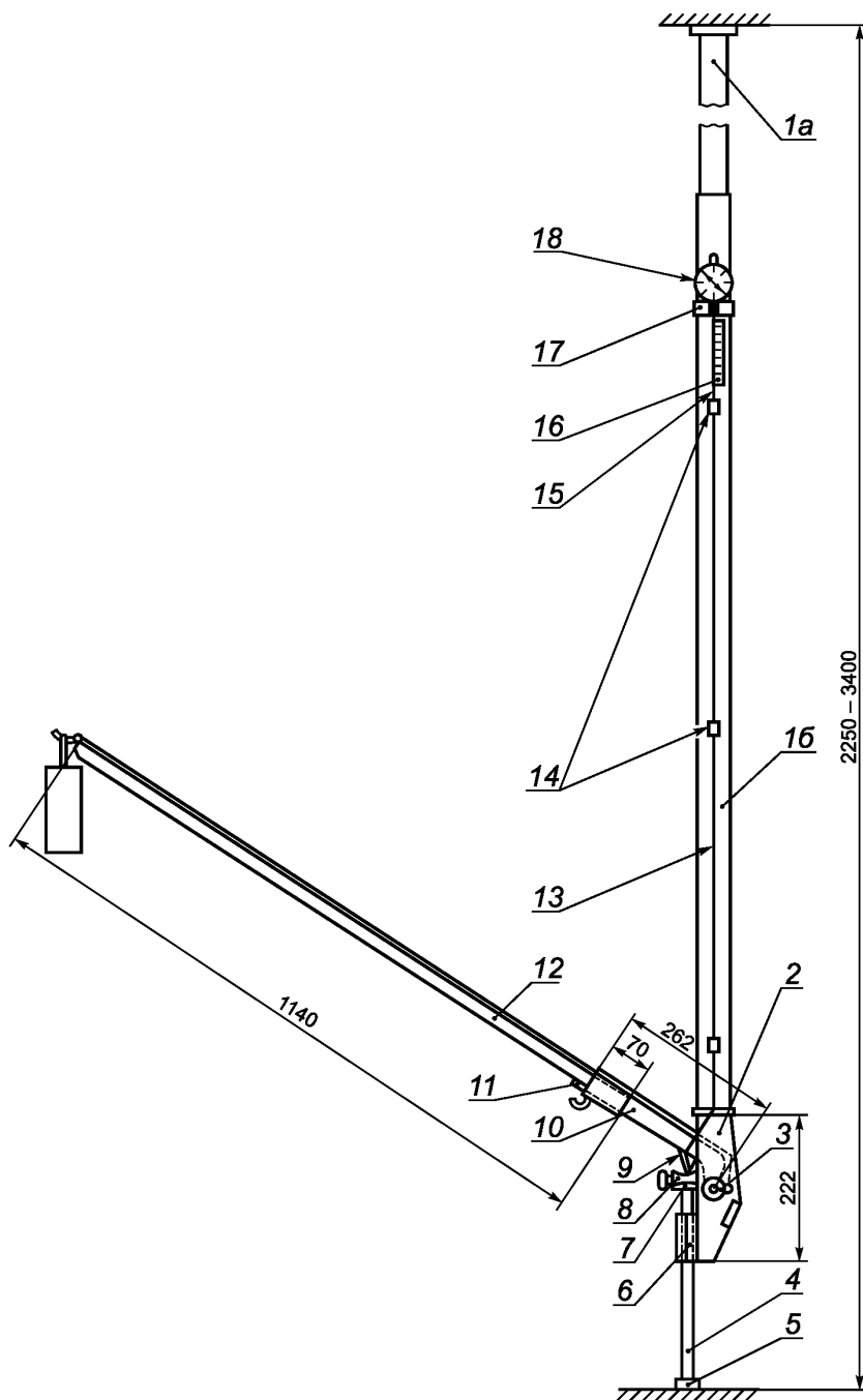
Рисунок 1 — Схема деформатора
