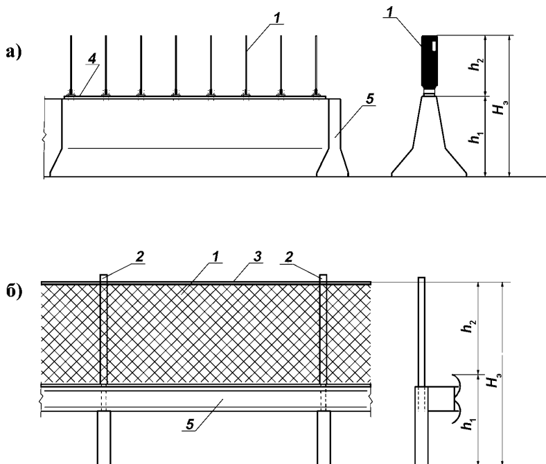
1 — затеняющий элемент; 2 — стойки; 3 — рейки; 4 — опора; 5 — основание (ограждение барьерного или парапетного типа); h_1 — высота ограждения; h_2 — высота затемняющего элемента; H_3 — эффективная высота экрана
