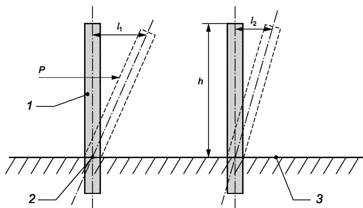
Рисунок 1 — Схема определения устойчивости сигнальных столбиков к воздействию ветровой нагрузки
