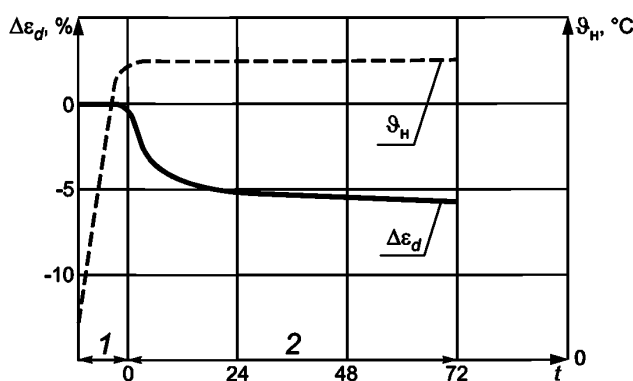
1 — период нагрева; 2 — период испытания; \Delta\varepsilon_d — изменение толщины, %; \Theta_n — температура нагревательной пластины, °С; t — время, ч
