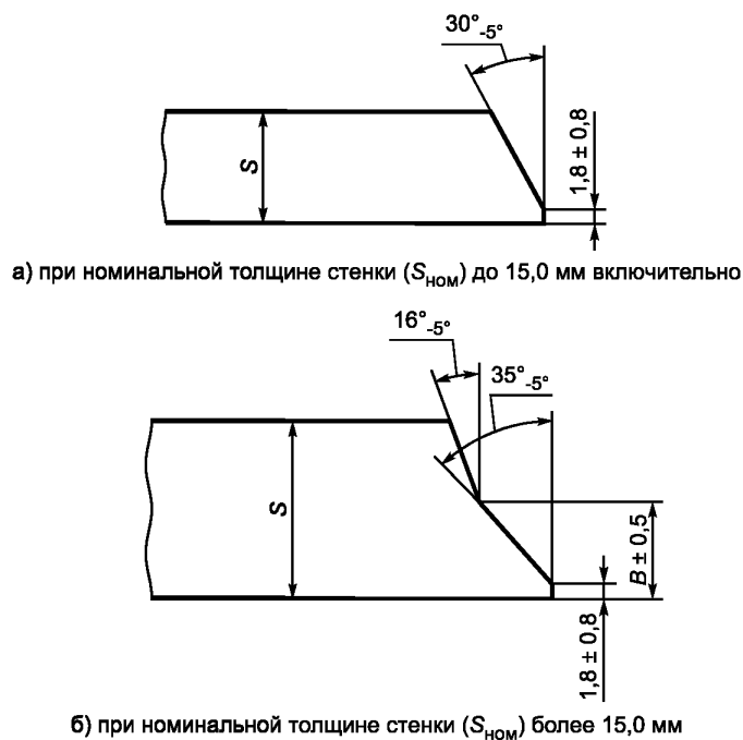
Рисунок 1 — Форма и размеры разделки торцов труб
