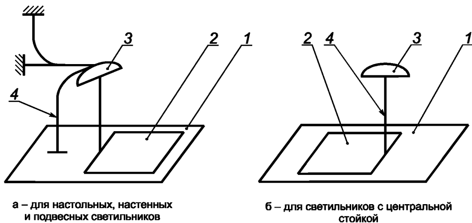
Рисунок 6 — Положение контрольной площади для измерения распределения освещенности
