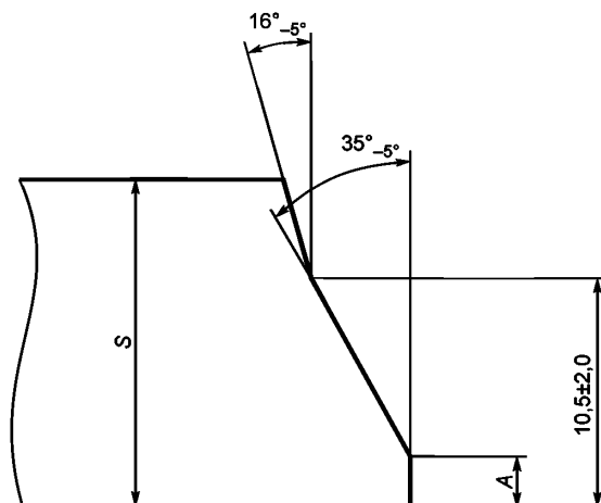
A — ширина торцевого притупления, S — толщина стенки
