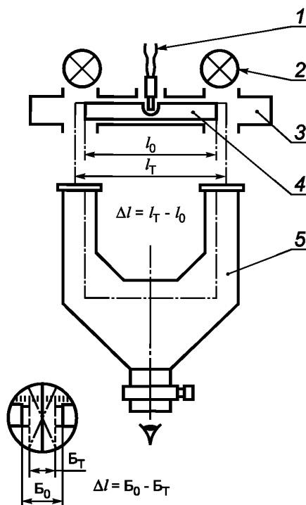
1 — термopара; 2 — осветитель; 3 — нагреватель; 4 — испытуемый образец; 5 — микроскоп-компаратор
